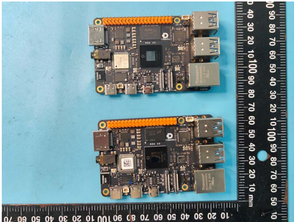
RDK X5 8G
