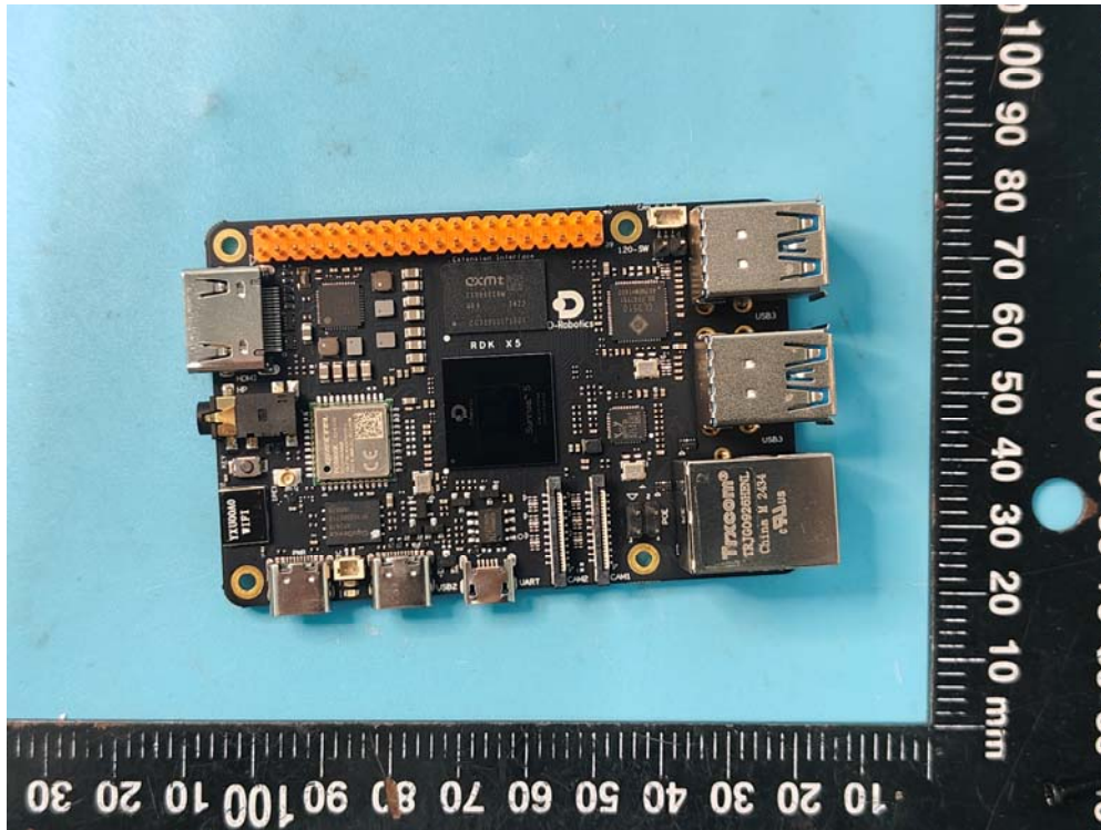
RDk X5 4G
