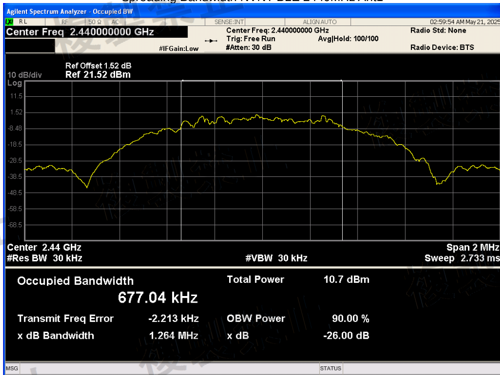
Spreading Bandwidth NVNT BLE 2440MHz Ant1
