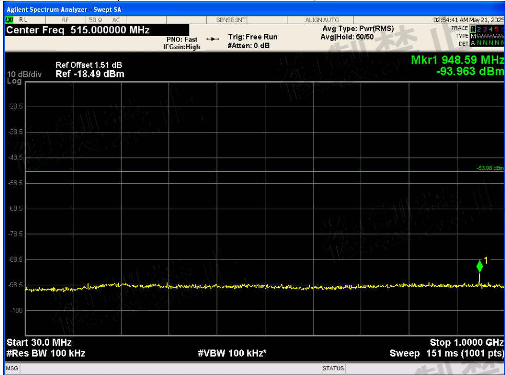
Rx. Spurious NVNT BLE 2402MHz Ant1 @ 30MHz-1000MHz
