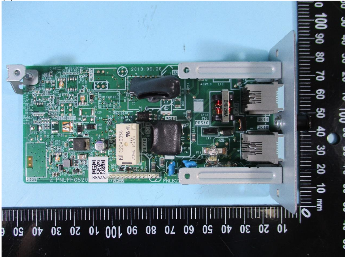
機板照片
