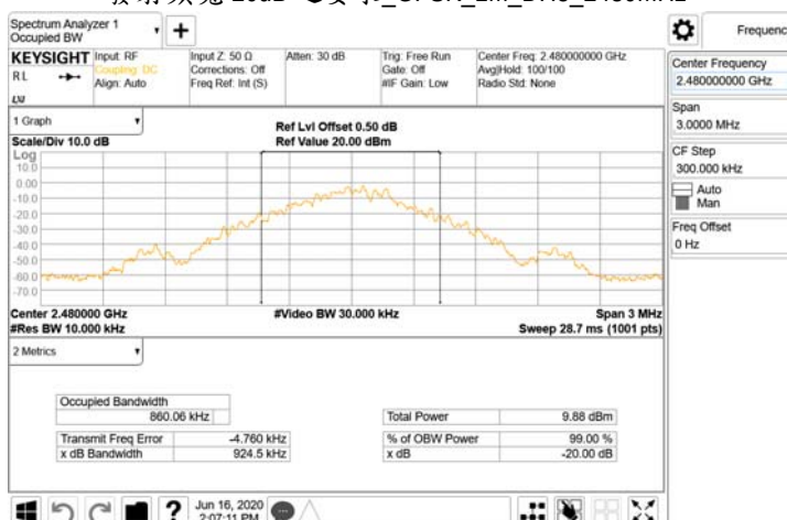
發射頻寬 20dB 之要求_GFSK_1M_DH5_2480MHz
