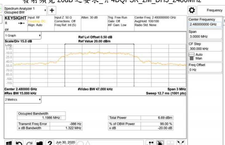
發射頻寬 20dB 之要求_π 4DQPSK_2M_DH5_2480MHz
