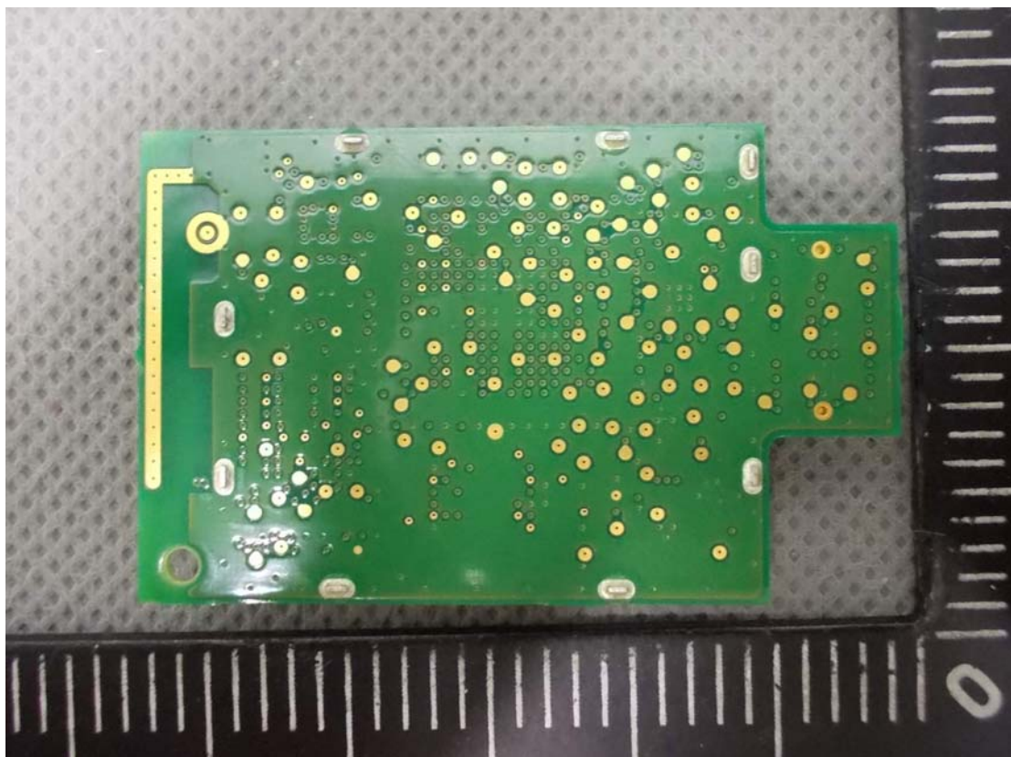
Module
