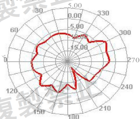
2450.000MHz E1
