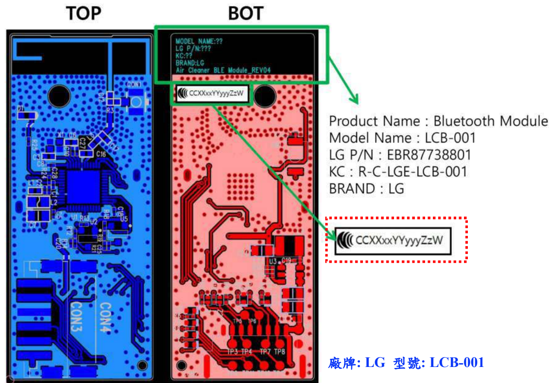
審驗合格標籤位置示意圖
