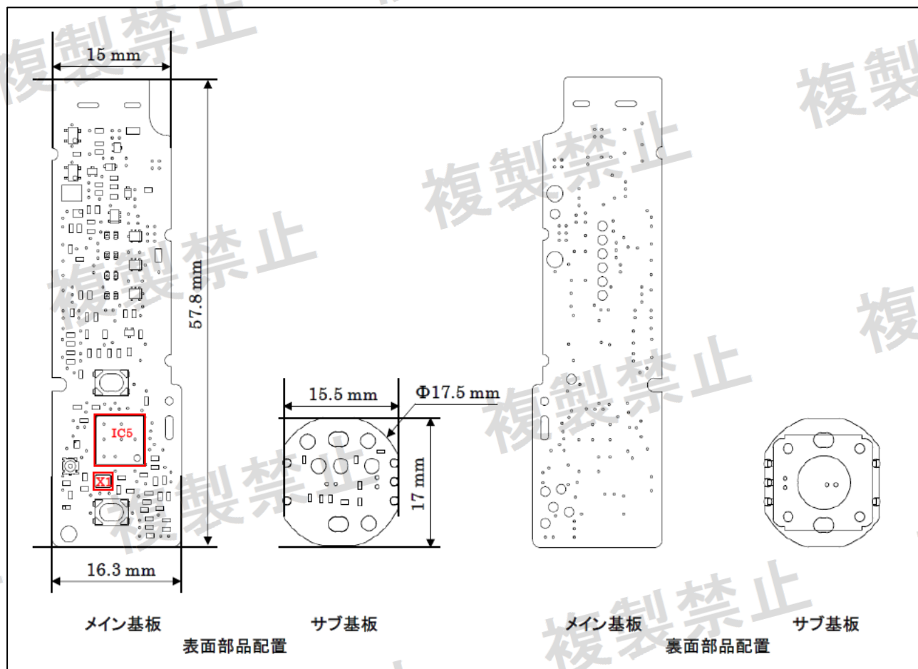
■基板部品配置図
