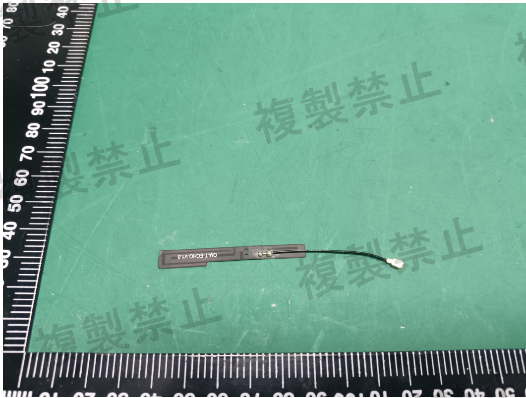
LoRa Antenna 2
