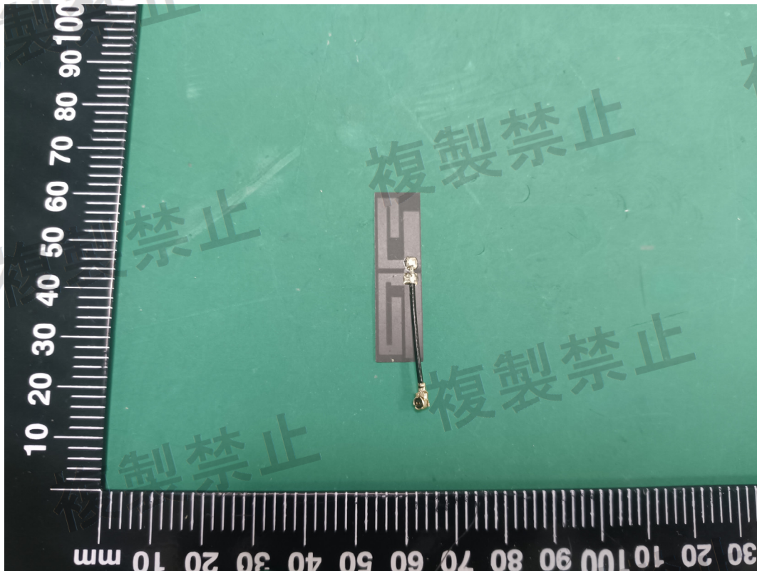
BLE Antenna
