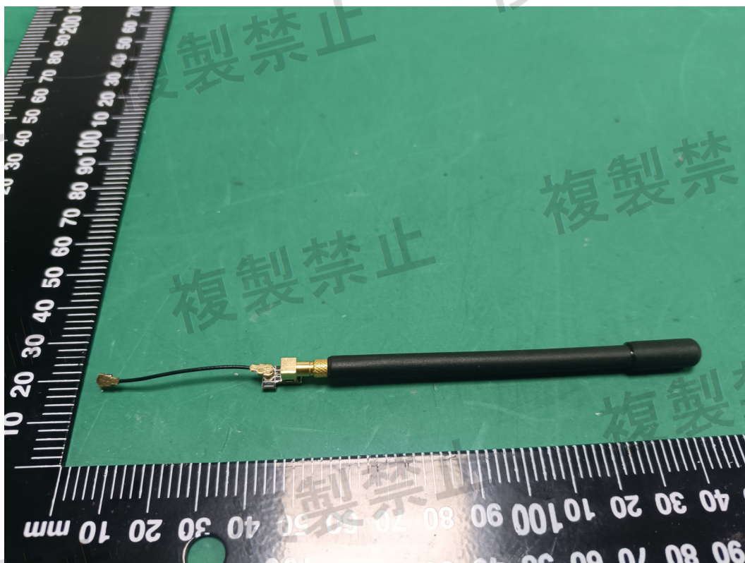
LoRa Antenna 1
