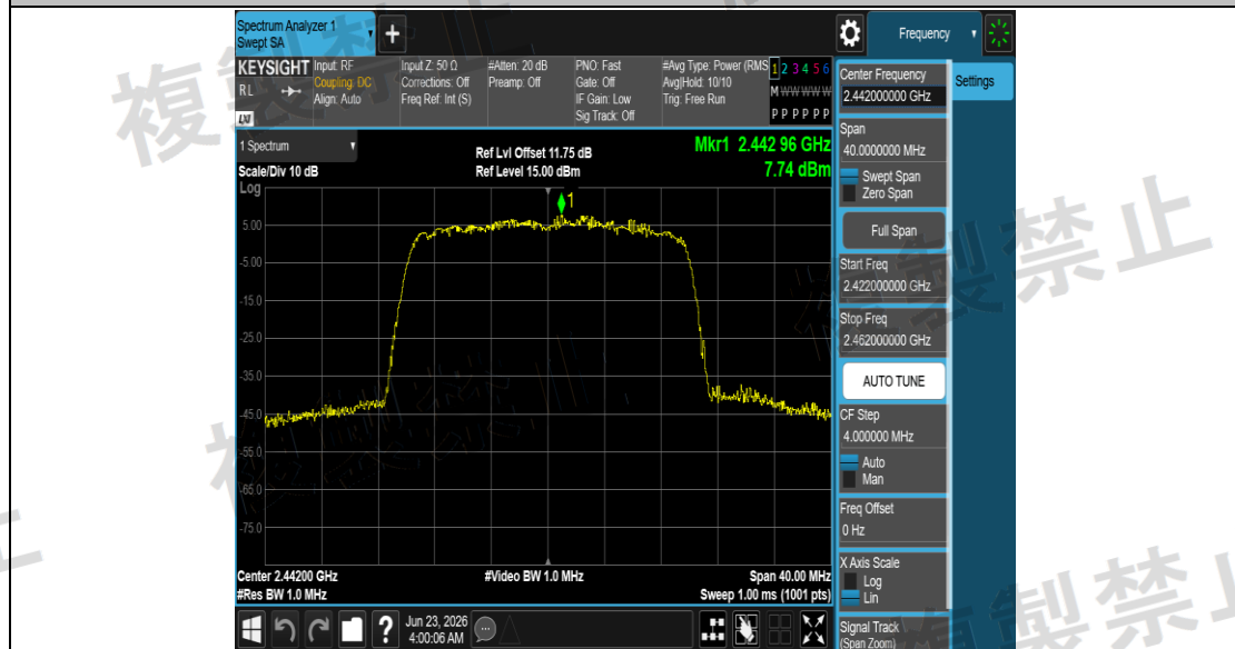
NTNV_11AX20SISO_Ant1_2442
