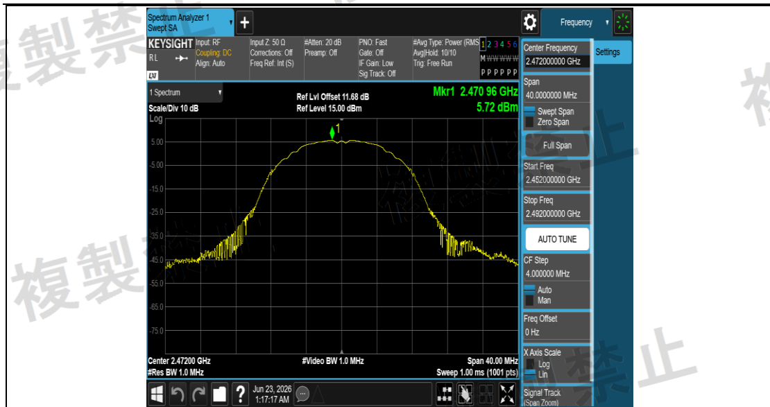
NTVN_11B_Ant1_2472
