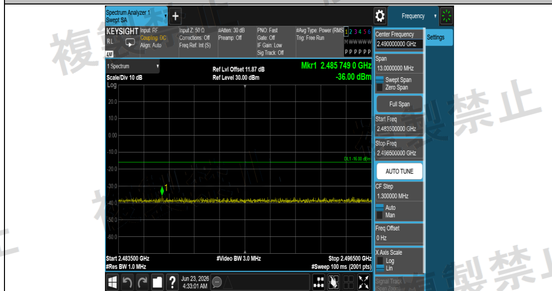
NTNV_11AX40SISO_Ant1_2422_2483.5~2496.5
