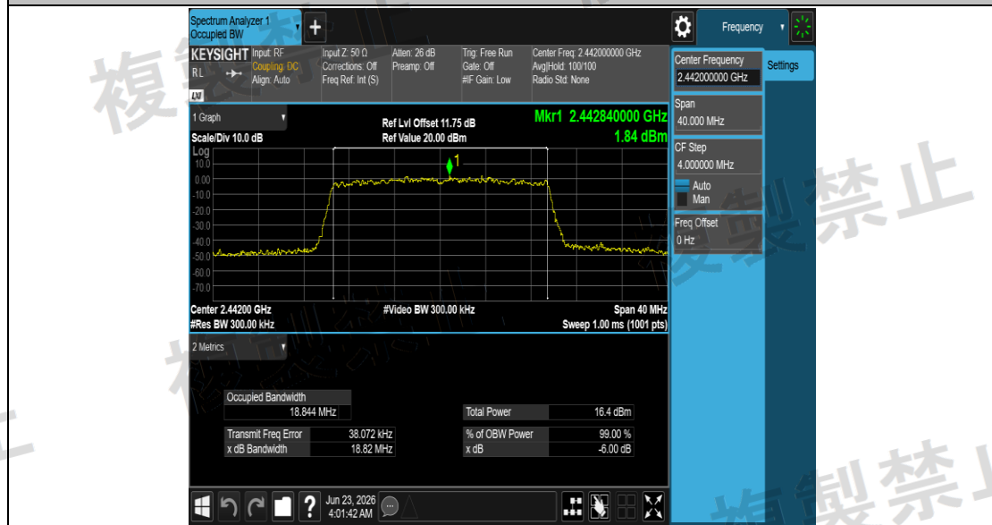
NTNV_11AX20SISO_Ant1_2442
