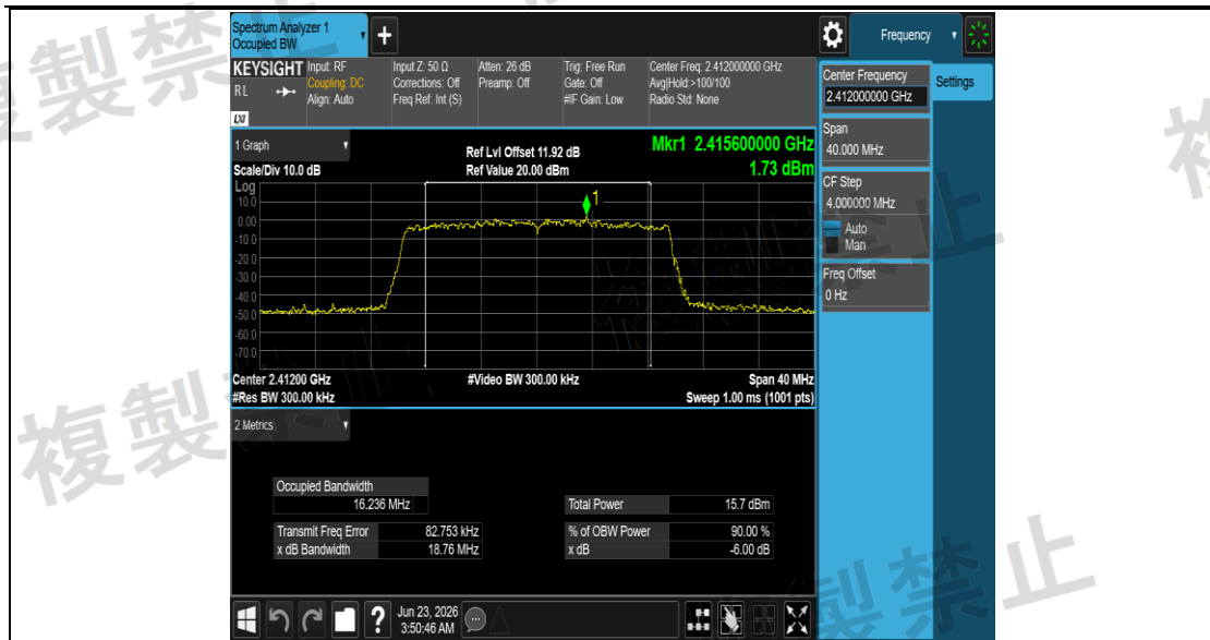
NTNV_11AX20SISO_Ant1_2412
