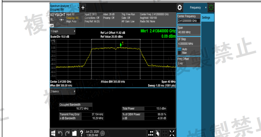
NTNV_11G_Ant1_2412
