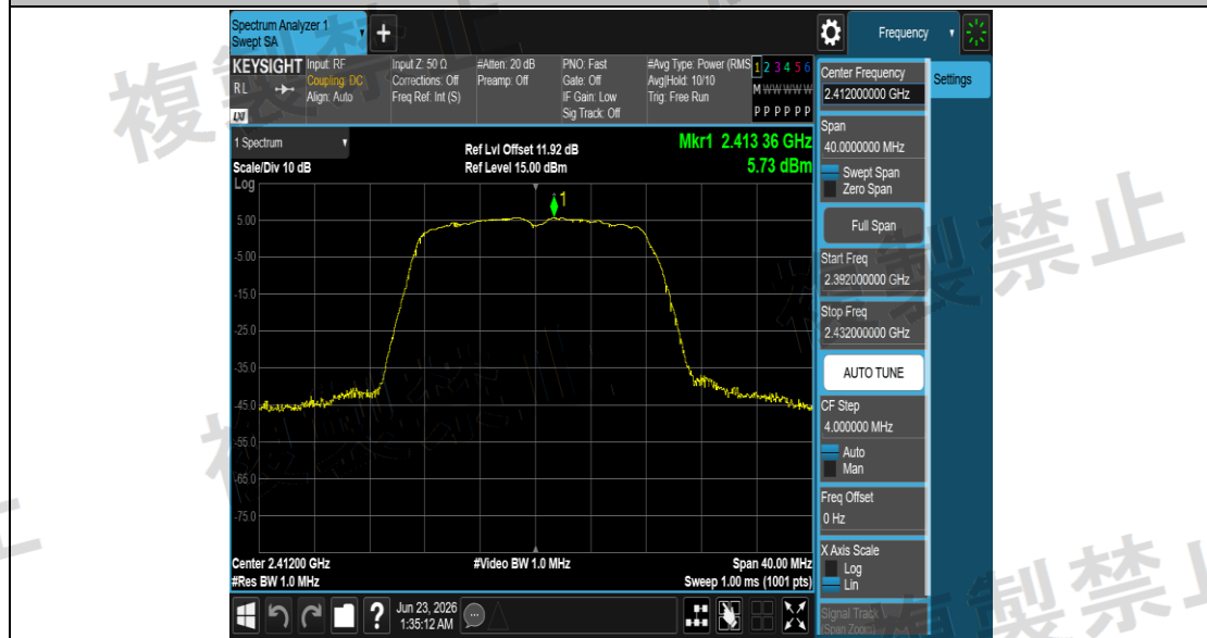
NTVN_11G_Ant1_2412
