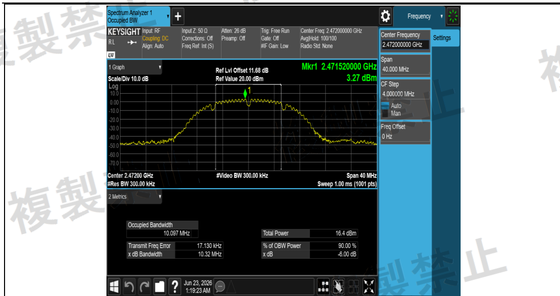
NTNV_11B_Ant1_2472
