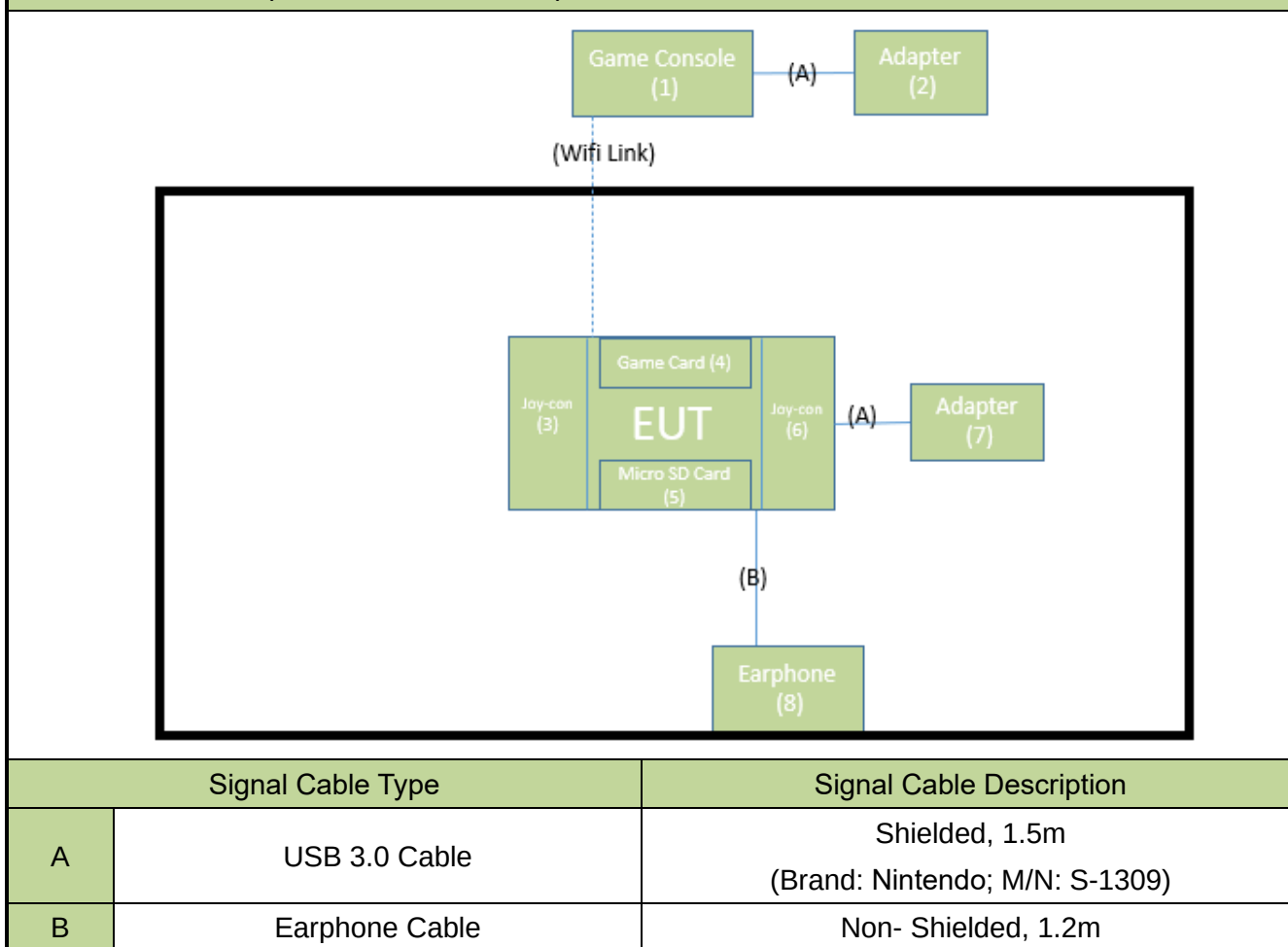
待測物測試配置圖 (Normal Mode / Mode5)
