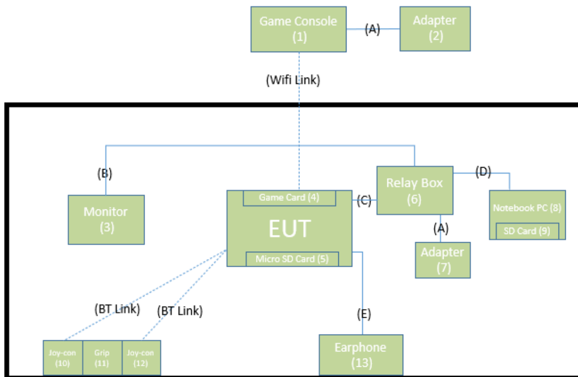
待測物測試配置圖 (Normal Mode / Mode6)
