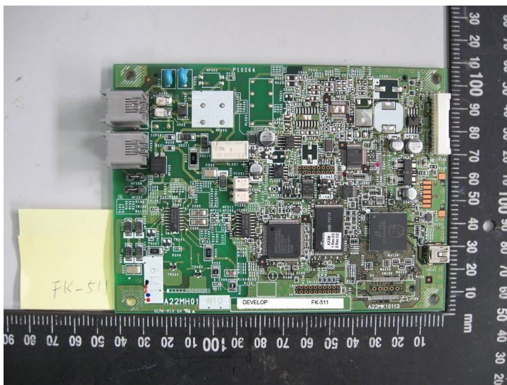
圖 6、傳真卡(廠家/型號: DEVELOP /FK-511)零件面 (適用機種: 廠牌:DEVELOP / 型號: ineo+ 554、ineo+ 454、DEVELOP ineo+ 554、DEVELOP ineo+ 454)
