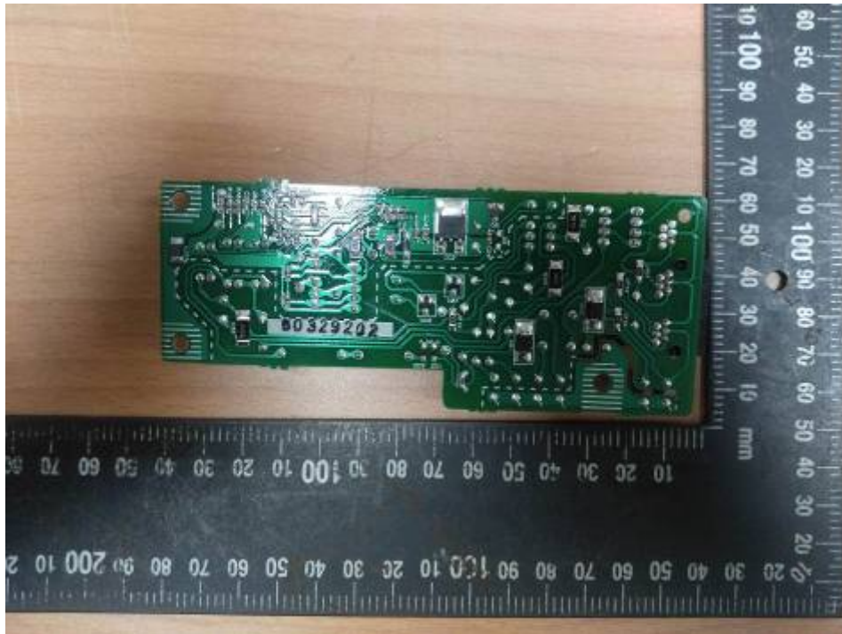
圖 6、NCU Unit 銅軌面
