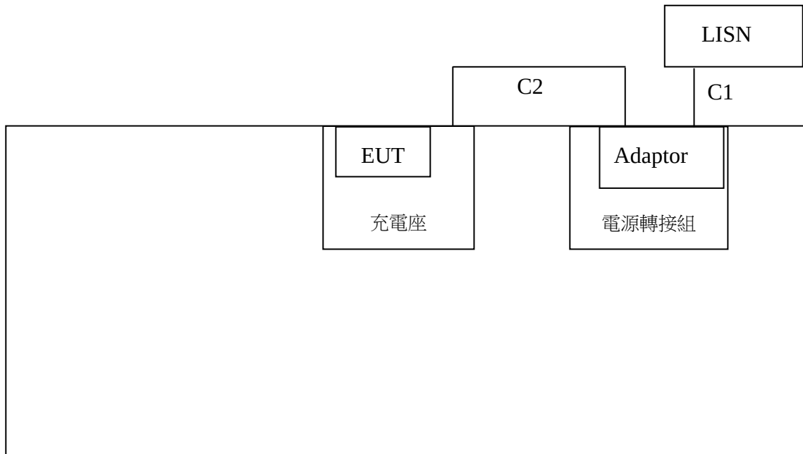
圖(一) 電源傳導受測系統連接圖
