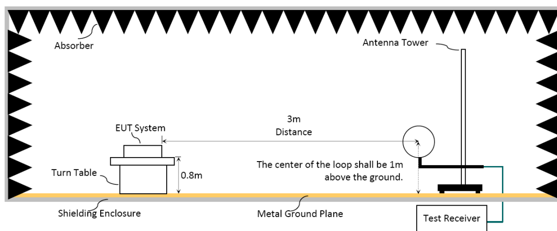
圖 2: 量測頻率於 9kHz-30MHz 之測試配置(3m Semi Anechoic Chamber)
