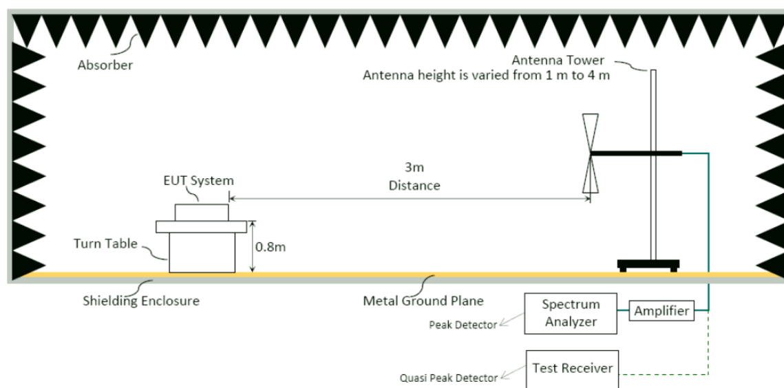
圖 3: 量測頻率於 30MHz-1GHz 之測試配置 3m Semi Anechoic Chamber)
