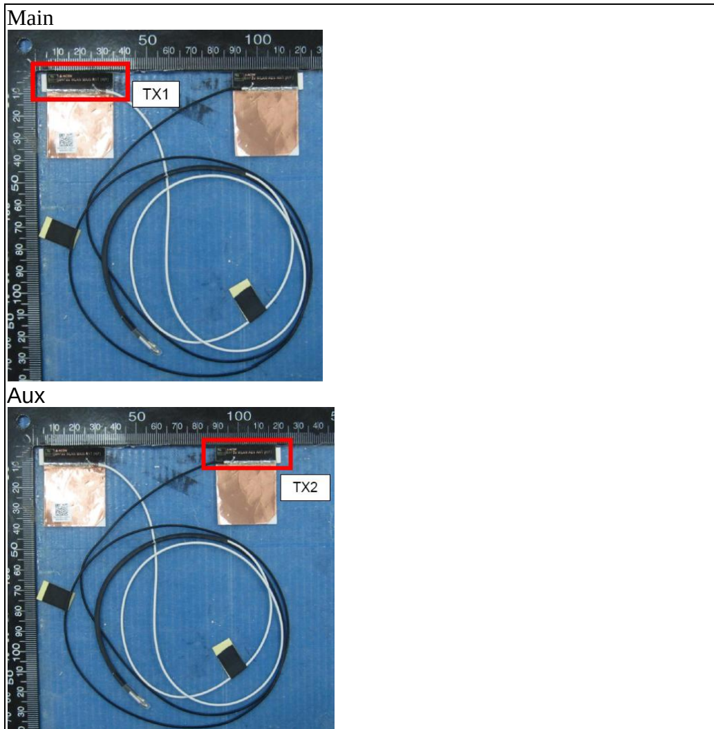
Antenna 11_ ANP6Y-200029(MAIN), ANP6Y-200029(AUX), ACON , 2016/8/22
