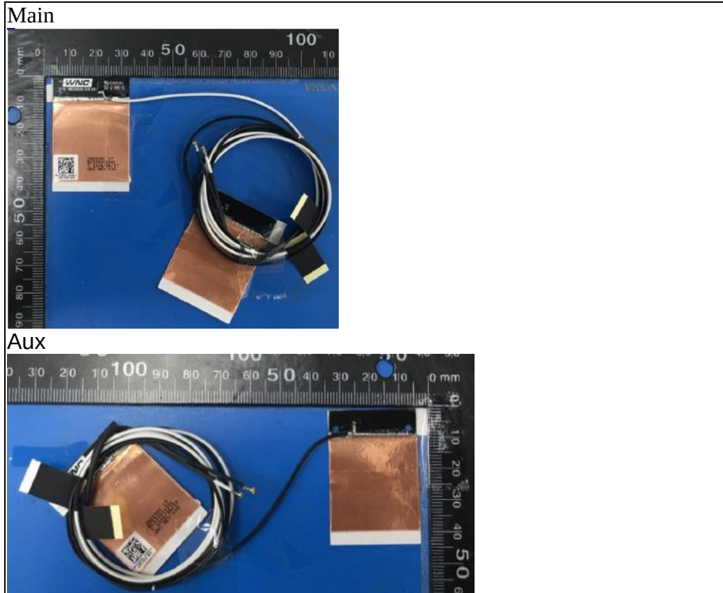
Antenna 11_ ANP6Y-200029(MAIN), ANP6Y-200029(AUX), ACON , 2016/8/22
