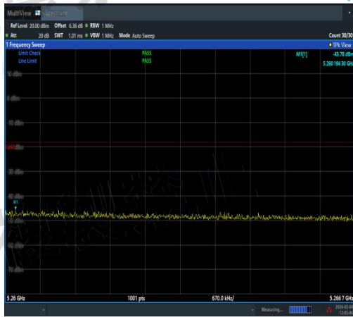
NTVN-11AX20MIMO-Ant1-5240-5260~5266.7-P ASS
