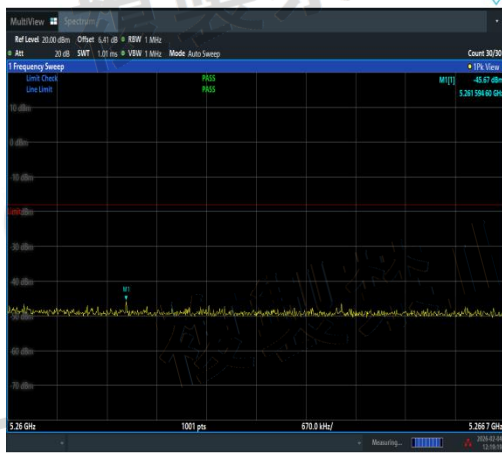
NTVN-11AX20MIMO-Ant3-5240-5260~5266.7-P ASS
