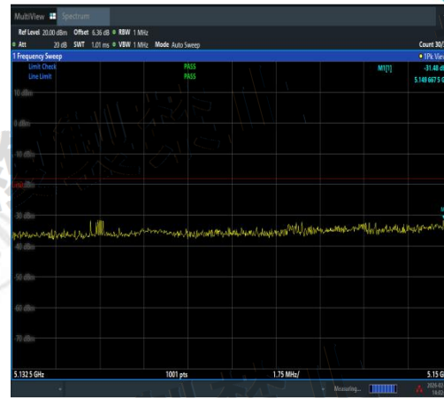
NTNV-11AX80SISO-Ant1-5210-5132.5~5150-PA SS
