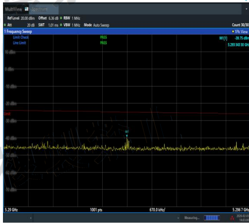
NTNV-11AX80SISO-Ant1-5210-5290~5296.7-PA
