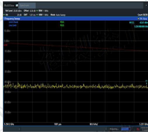
NTVN-11AX20MIMO-Ant1-5220-5250.2~5251-P ASS
