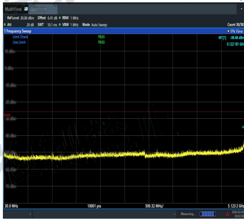
NTNV-11AX80SISO-Ant3-5210-30~5123.2-PASS
