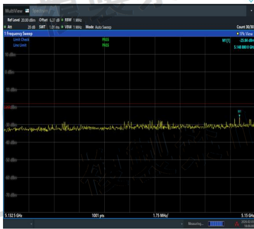
NTNV-11AX80SISO-Ant2-5210-5132.5~5150-PA SS
