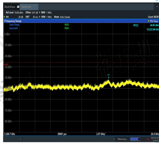
NTVN-11AX20MIMO-Ant1-5240-5266.7~26000-P ASS
