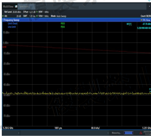
NTVN-11AX20MIMO-Ant1-5180-5250.2~5251-P ASS
