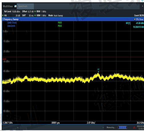
NTVN-11AX20MIMO-Ant3-5240-5260~5266.7-P ASS
