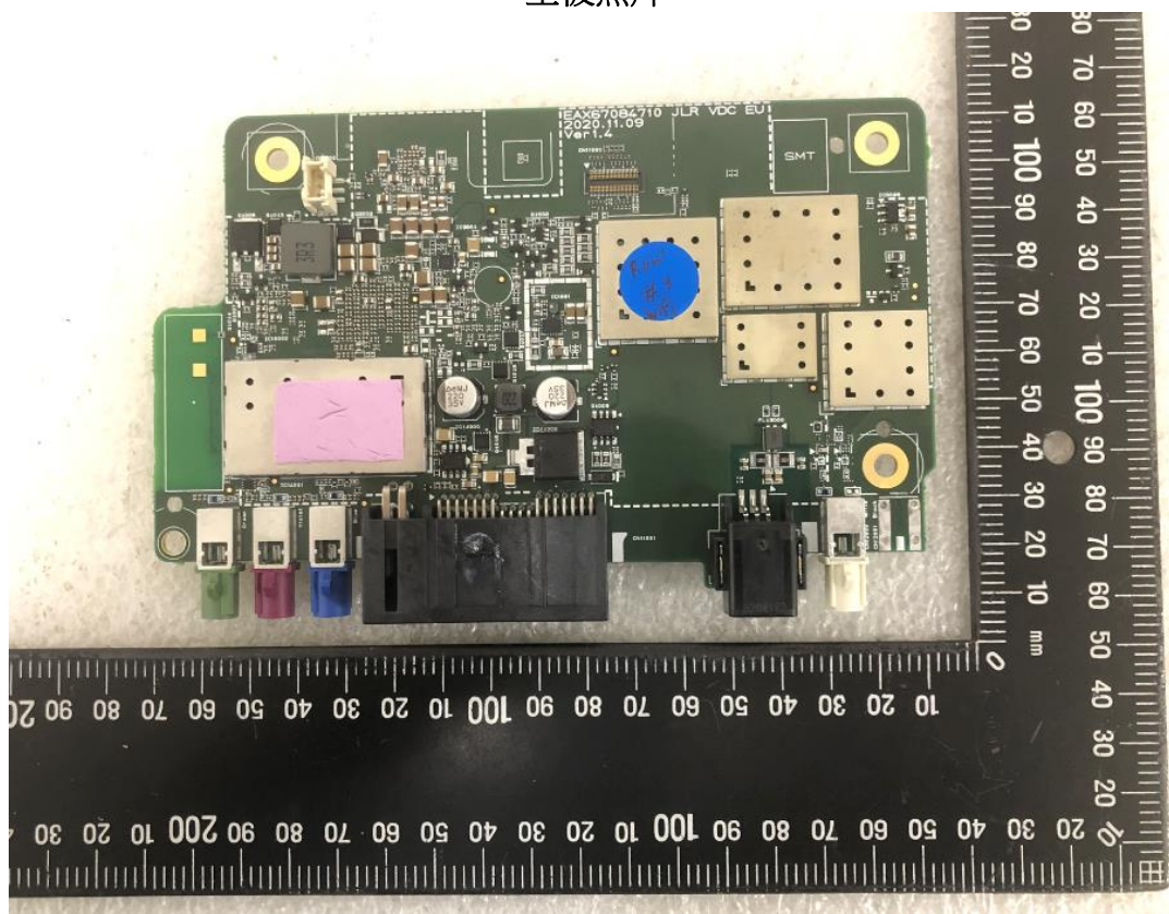
主板照片
