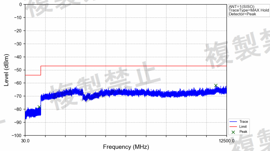
1M_2402MHz_Ant1_NTLV
