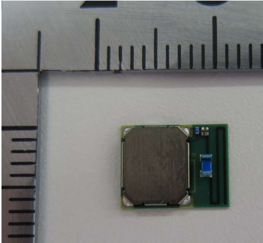
BLE Module (WM500)
