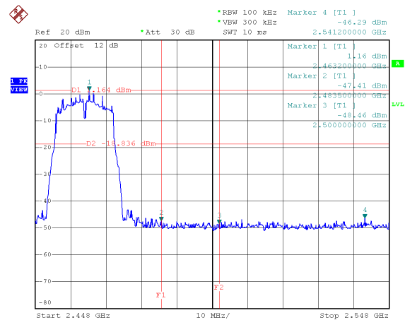
上邊緣頻帶-CH11
