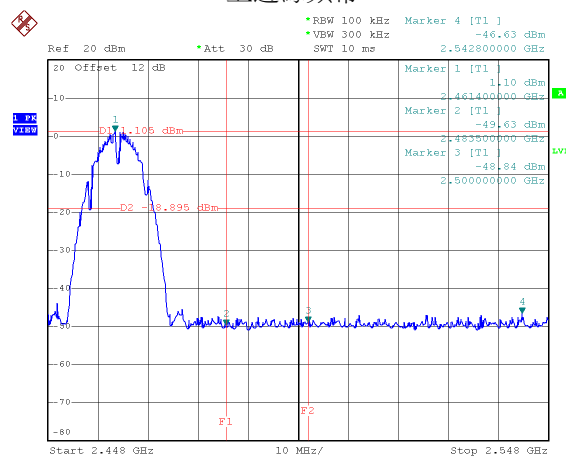
上邊緣頻帶-CH11
