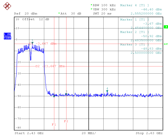
上邊緣頻帶-CH09
