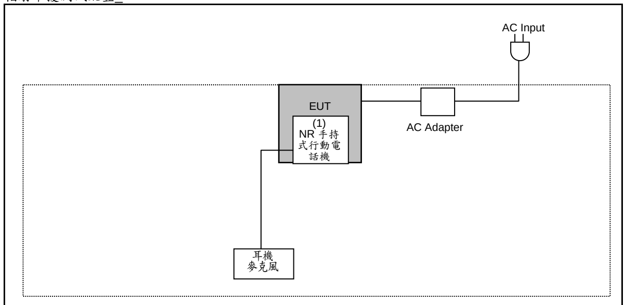
輻射干擾測試配置_TX
