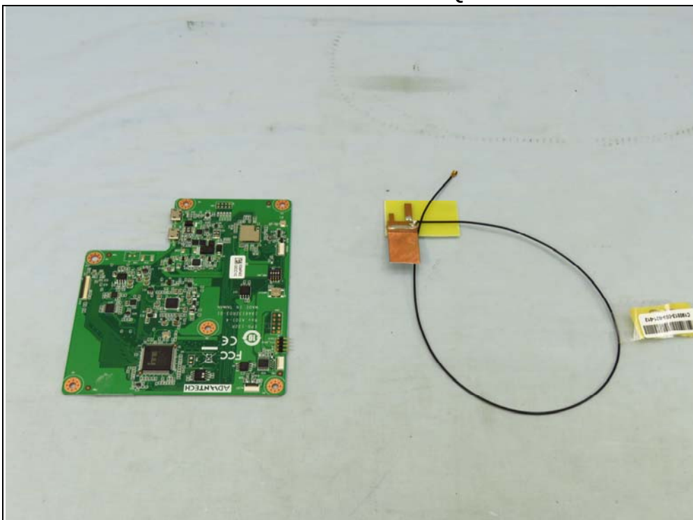
EUT with antenna P/N: AJMQ1J-B0007
