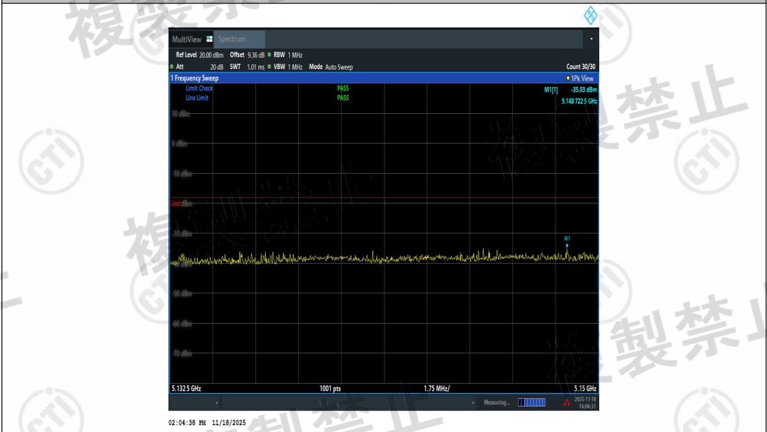
NTNV-11AC80SISO-Ant1-5210-5132.5~5150-PASS
