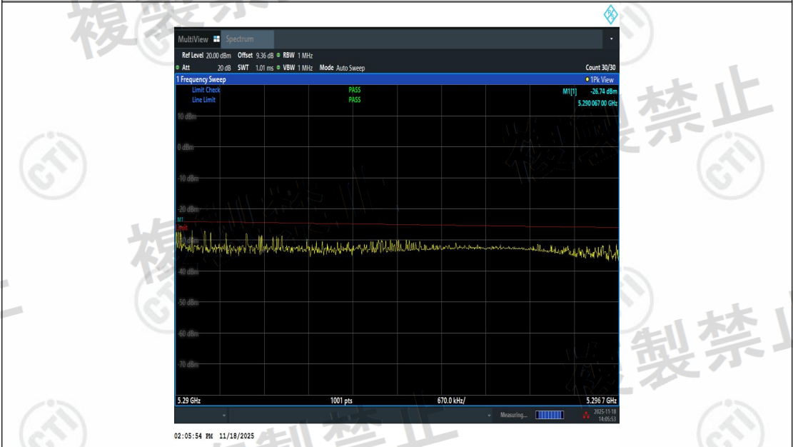
NTNV-11AC80SISO-Ant1-5210-5290~5296.7-See table below
