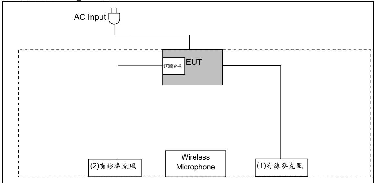
電源傳導干擾測試配置_With 隨身碟
