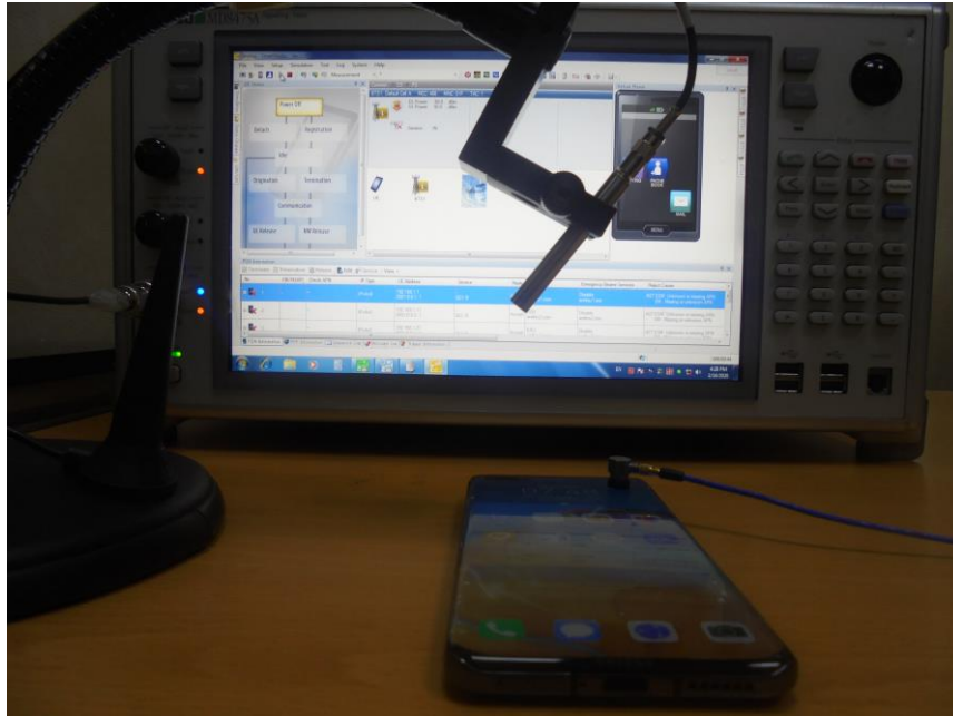
公眾告警廣播 SETUP 照
