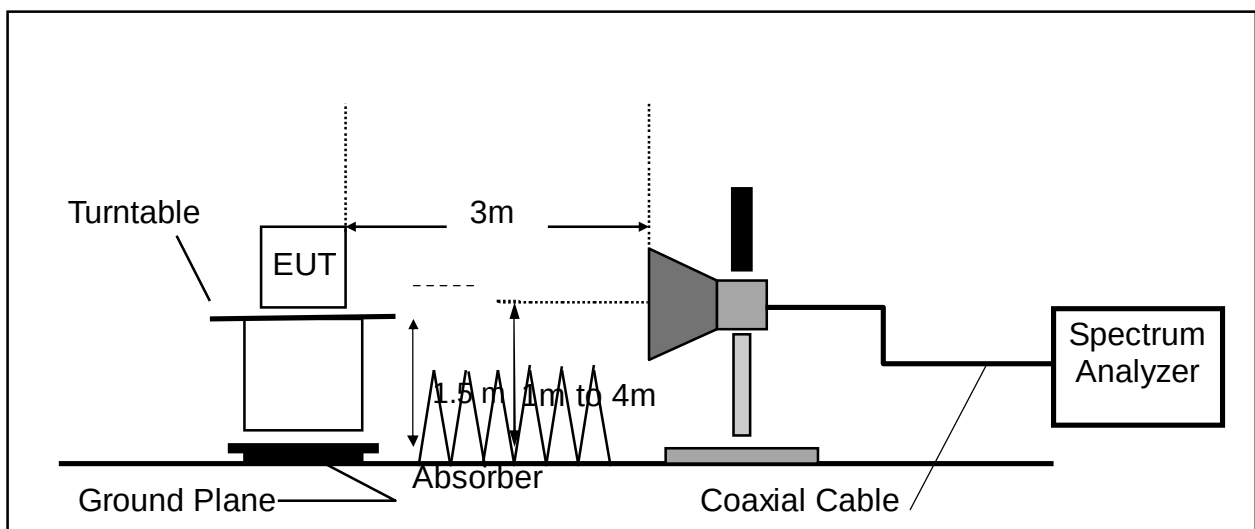
(b) 輻射量測配置圖:
