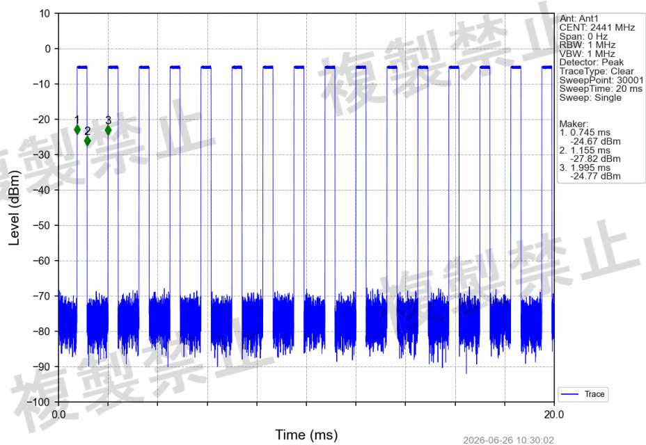
GFSK DH3 2441MHz Ant1 NTN
