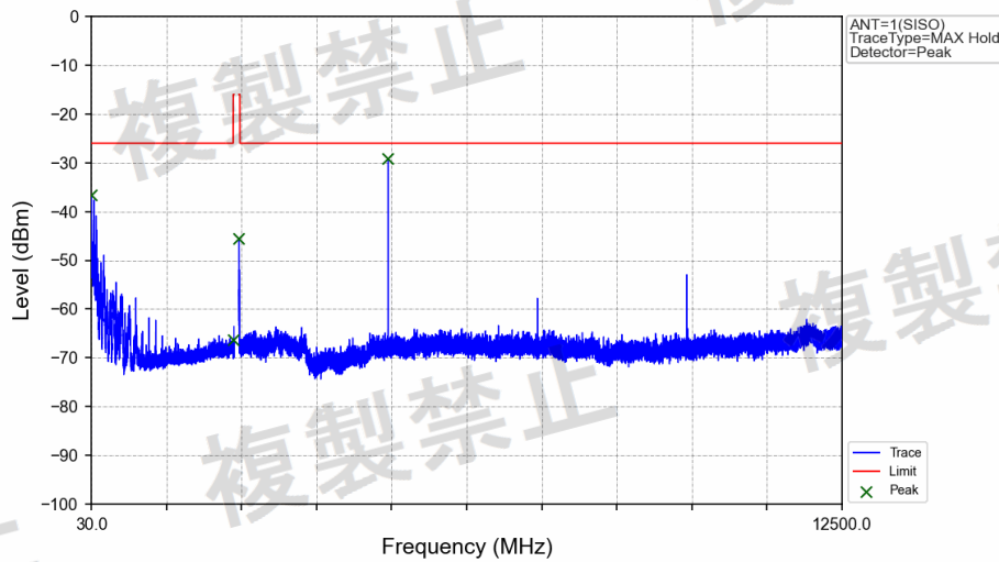
8DPSK 3DH5 2480MHz Ant1 NTN
