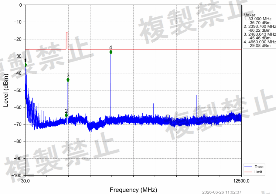
8DPSK 3DH5 2480MHz Ant1 NTN
