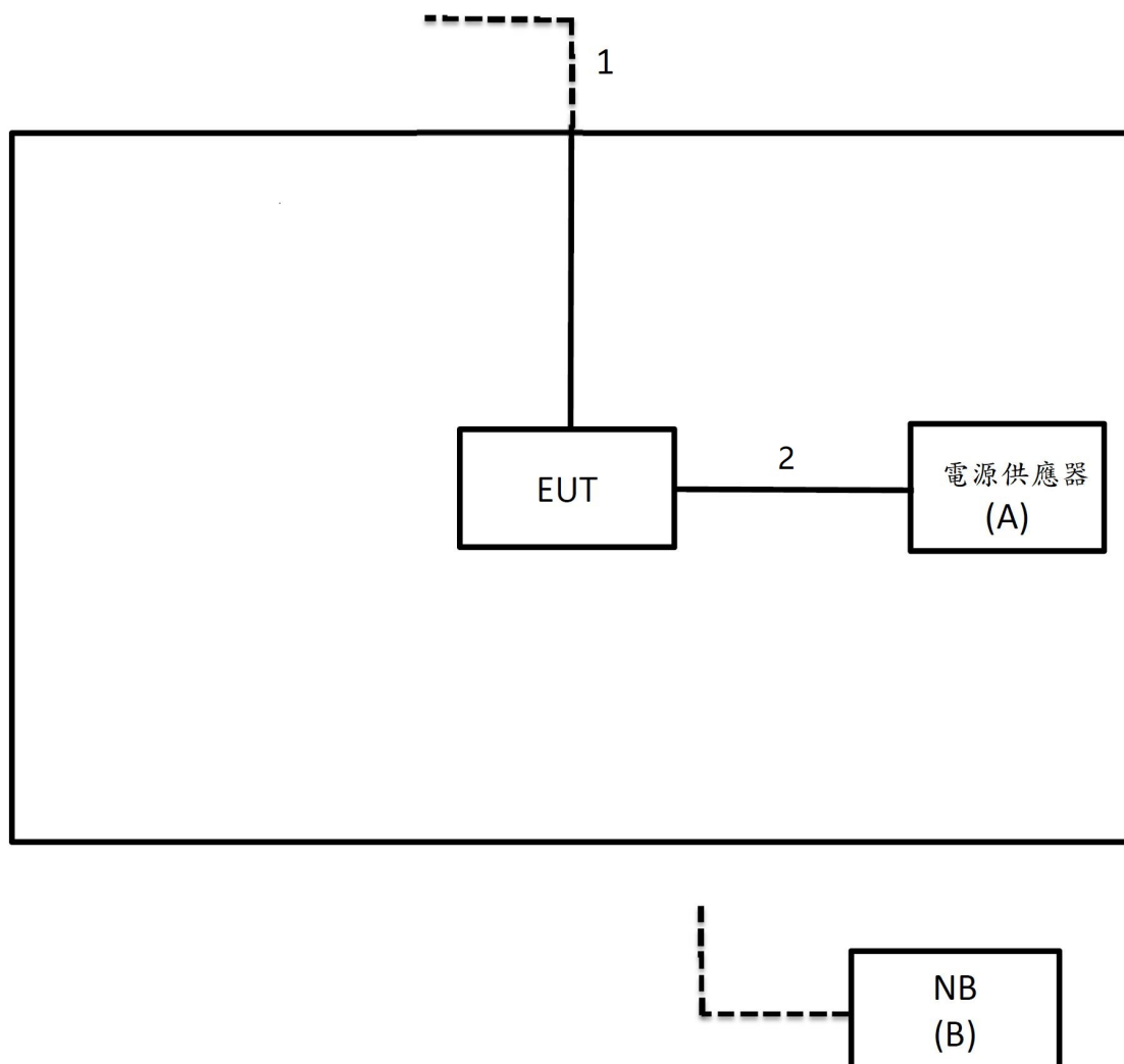
圖（一）、測試系統組成示意圖
