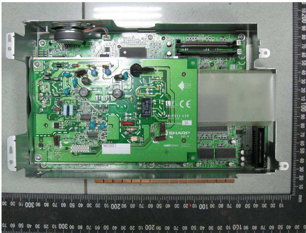
相片二：傳真盒內部(2)(廠牌：SHARP 型號：MX-FX10)
