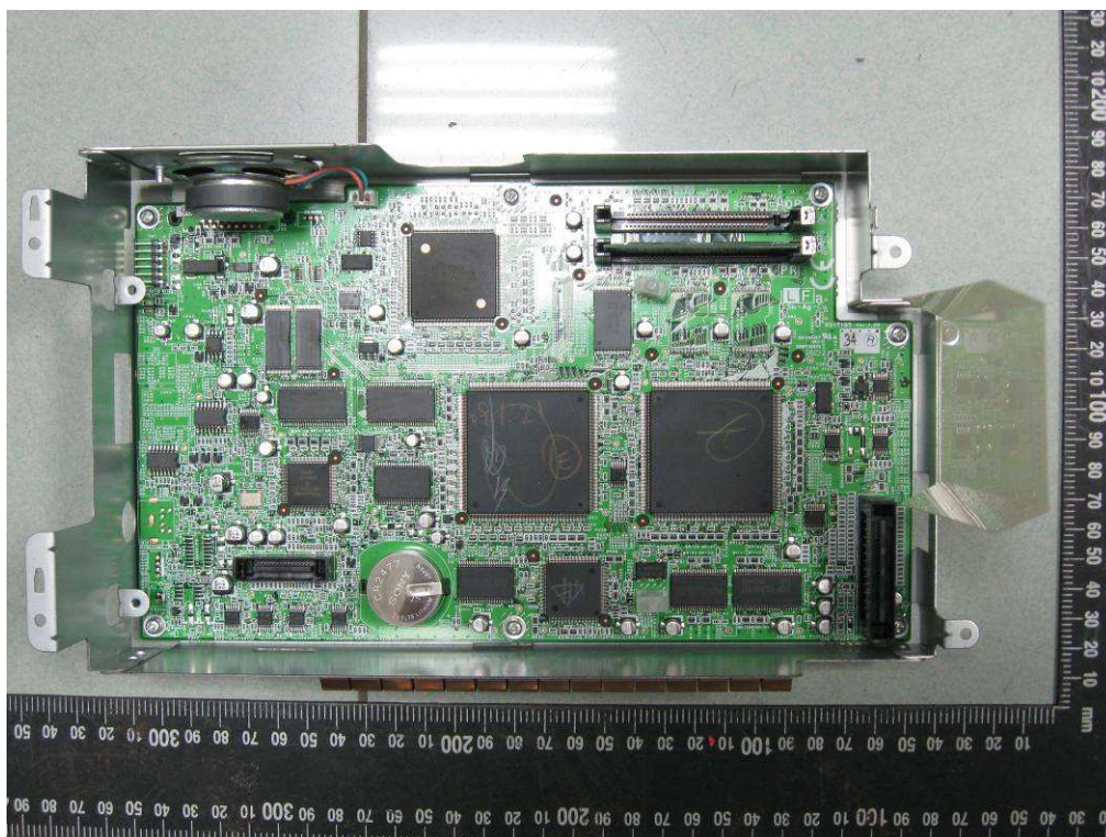
相片二：傳真盒內部(2)(廠牌：SHARP 型號：MX-FX10)
