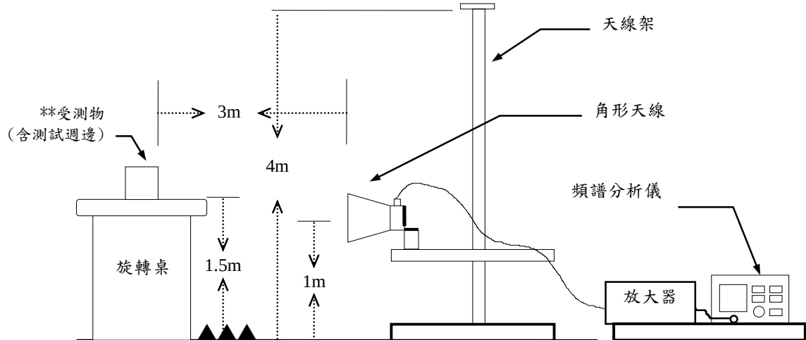
圖 3：量測頻率1GHz以上之測試配置
