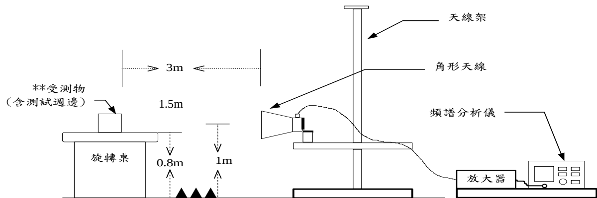
輻射量測配置圖
