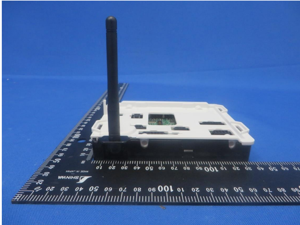
(5) 待測物照片
