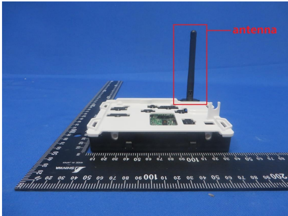
(7) 待測物照片
