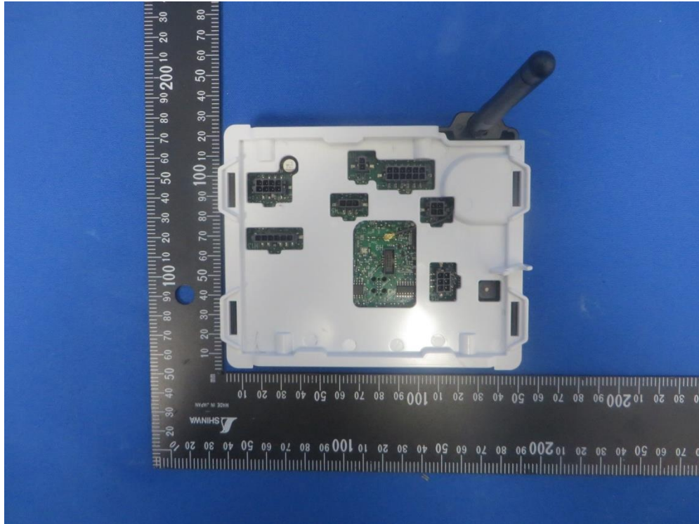
(1) 待測物照片
