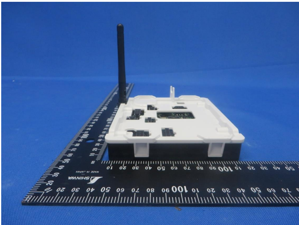
(6) 待測物照片
