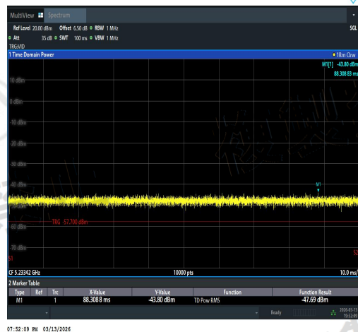
NTNV-11AX20MIMO-Ant1-5260-5233.3~5240-P ASS
