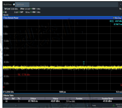
NTNV-11AX20MIMO-Ant2-5260-5233.3~5240-P ASS
