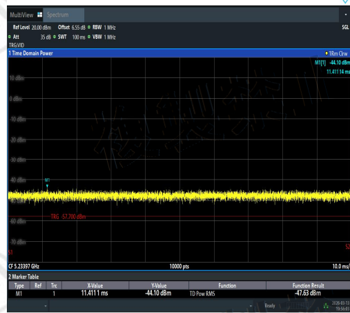
NTNV-11AX20MIMO-Ant3-5260-5233.3~5240-P ASS
