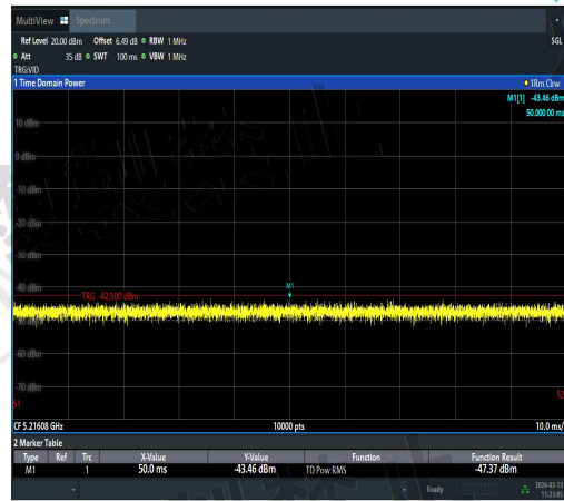
NTNV-11AC40SISO-Ant1-5270-30~5221.6-PAS
