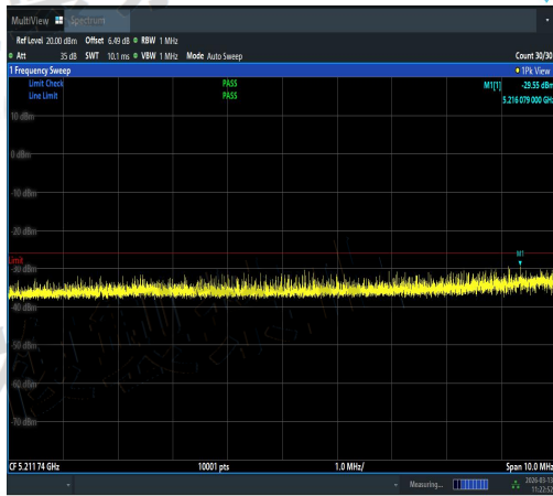
NTNV-11AC40SISO-Ant1-5270-30~5221.6-PAS
