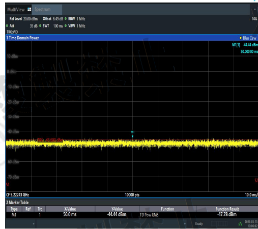
NTNV-11AC40MIMO-Ant3-5270-5221.6~5230-P ASS
