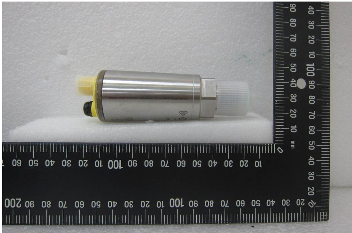
EUT 2 VEGABAR 28
