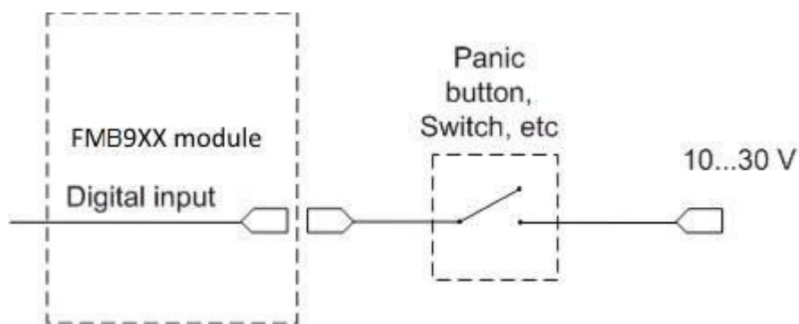
Рис. 5. Подключение тревожной кнопки
