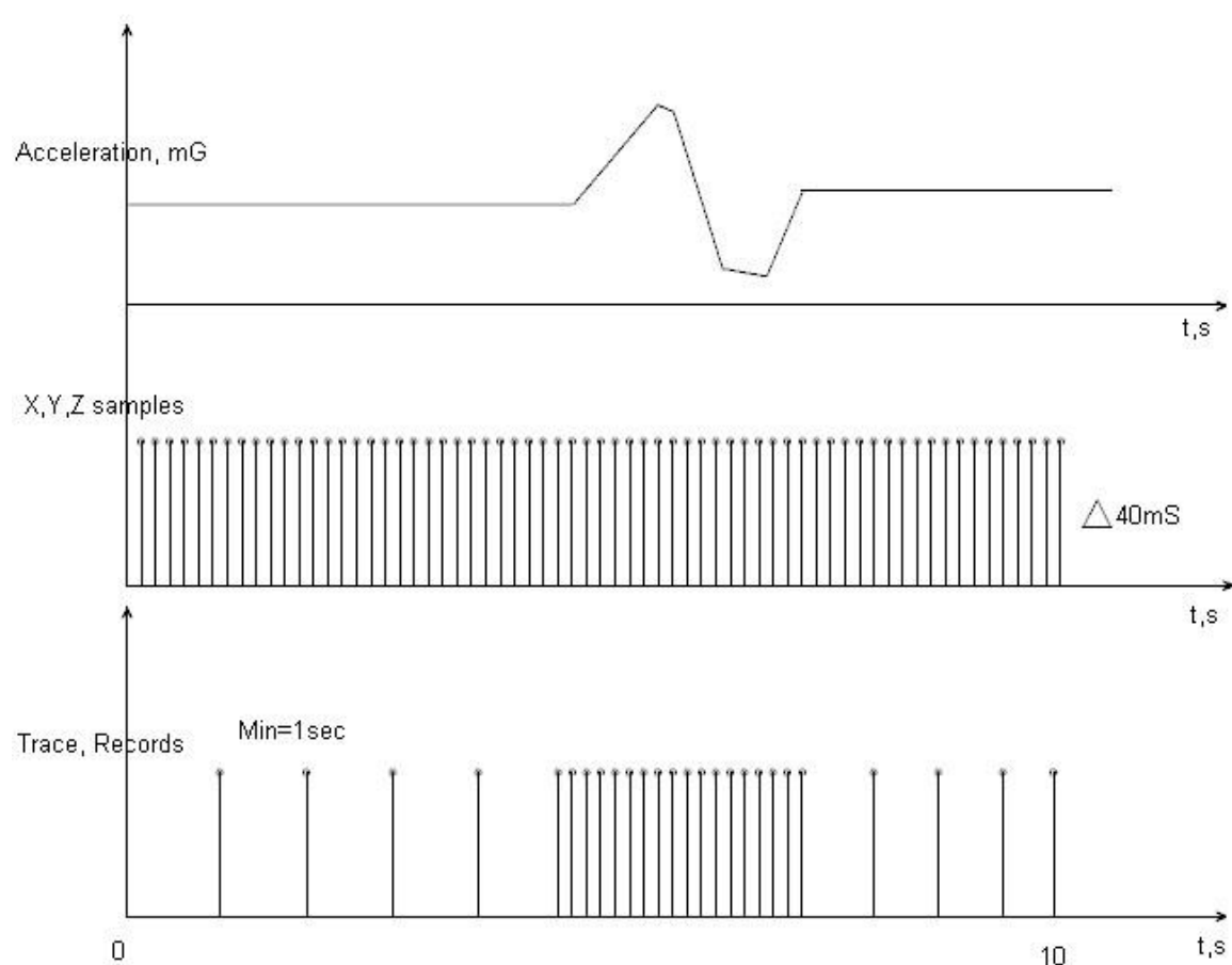
Рис. 10 Пример логики построения диаграммы аварии
