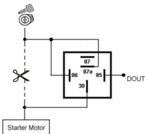
Рис.7 Подключение иммобилайзерного реле
