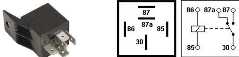
Рис. 8. Схема контактов автомобильного реле
