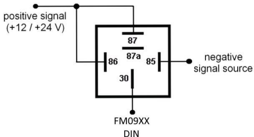
Рис. 6. Подключение инвертирующего реле
