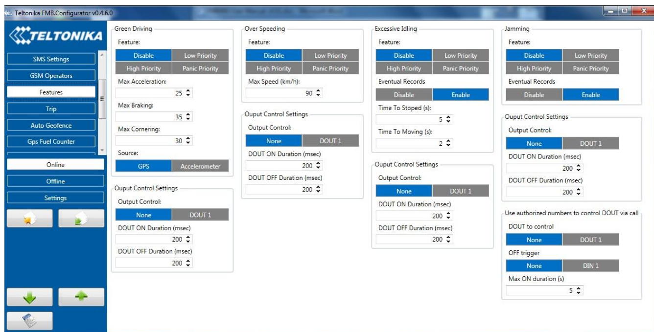
Рис.18 Настройка сценариев
