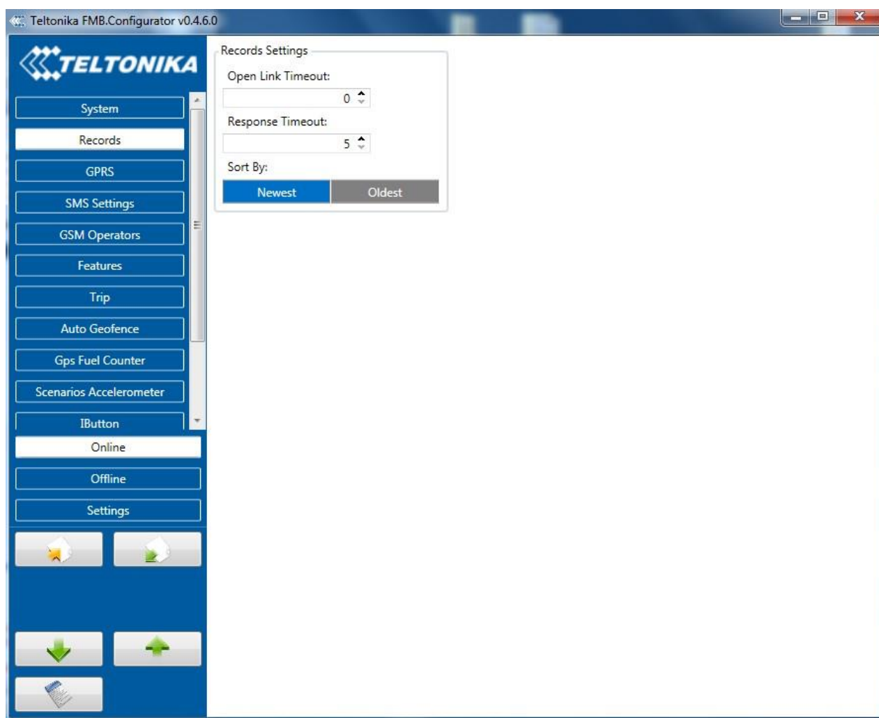
Рис. 12 Конфигурация записей
