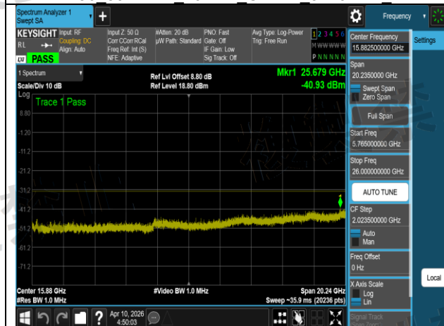
W56 802.11ax 20MHz Chain2 5500MHz 4
