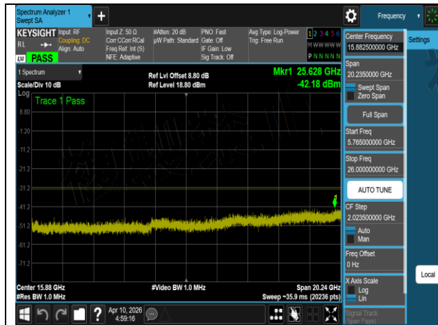
W56 802.11ax 20MHz Chain1 5600MHz 4
