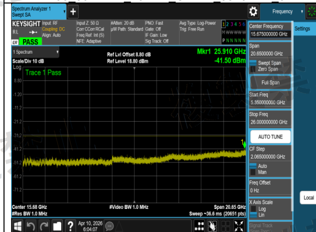
W53 802.11ax 20MHz Chain2 5260MHz 6
