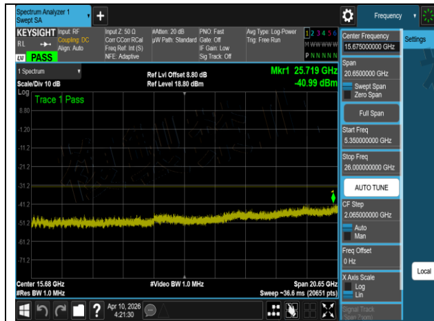
W53 802.11ax 20MHz Chain1 5300MHz 6
