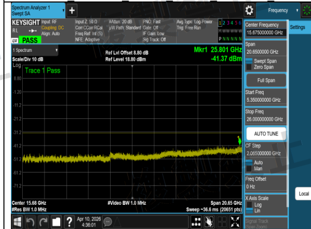
W53 802.11ax 20MHz Chain1 5320MHz 6
