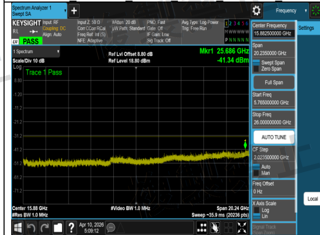
W56 802.11ax 20MHz Chain1 5720MHz 4
