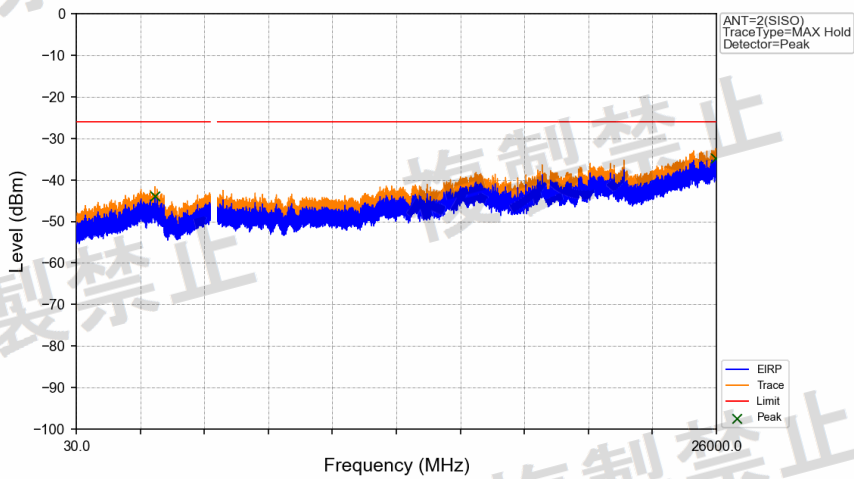
802.11a_MCH_5600MHz_Ant2_NTNV
