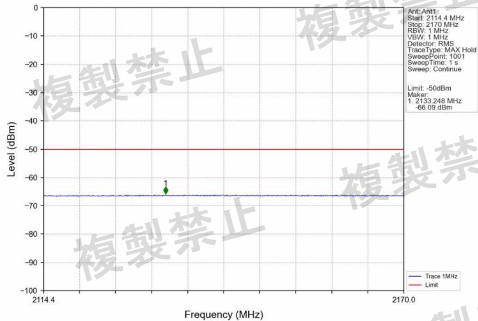
Band18_10MHz_QPSK_LCH_820MHz_RB_1_49_NTNV 17/25 2114.4-2170MHz Limit:-50
