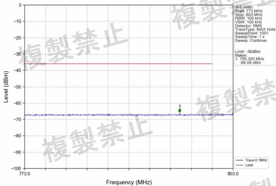
Band18_10MHz_QPSK_LCH_820MHz_RB_1_0_NTNV 10/25 773-803MHz Limit:-36
