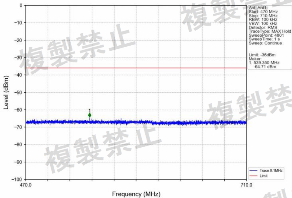
Band18_10MHz_QPSK_LCH_820MHz_RB_1_0_NTNV 8/25 470-710MHz Limit:-36
