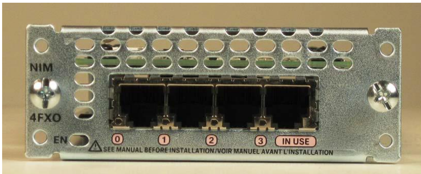
前視照
