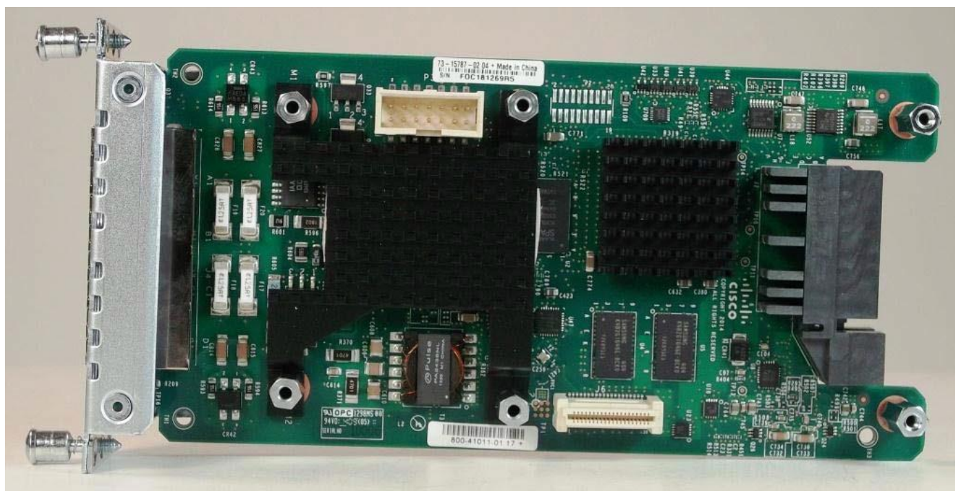
上視照
