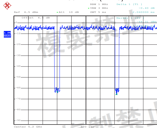
802.11ac(HT20)
