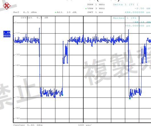
802.11ac(HT80)
