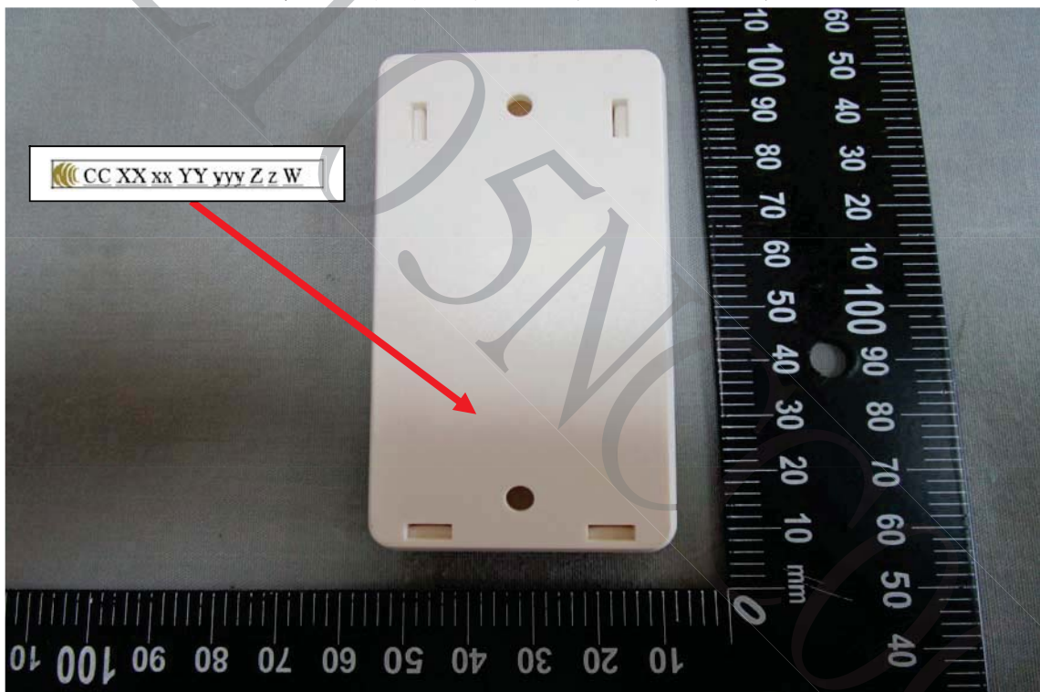
6) 待測物外觀底部照 (發射器)
