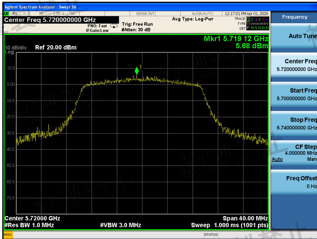
W56\Antenna Power Error\802.11ax HE20\1-5720-TX0-N
