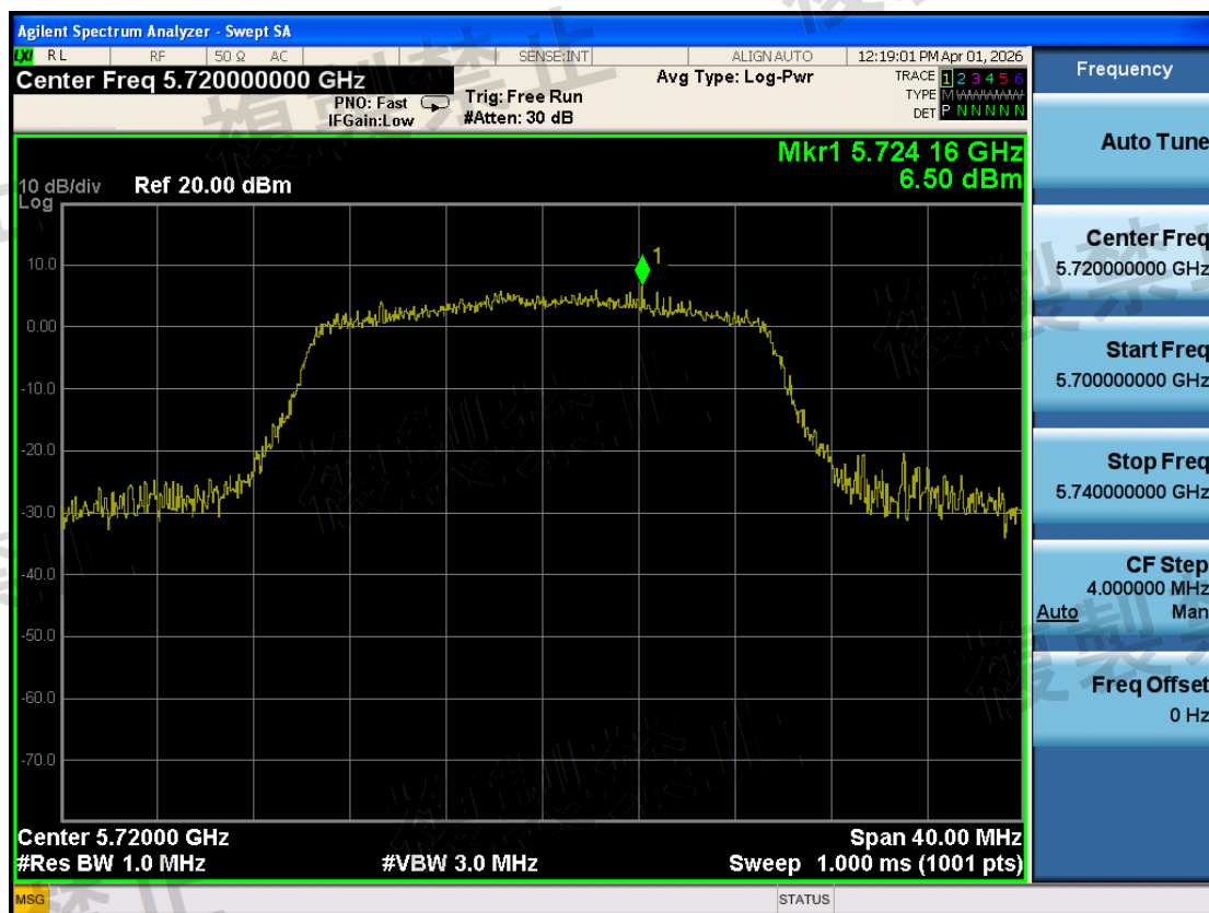
W56\Antenna Power Error\802.11ax HE20\1-5720-TX1-N
