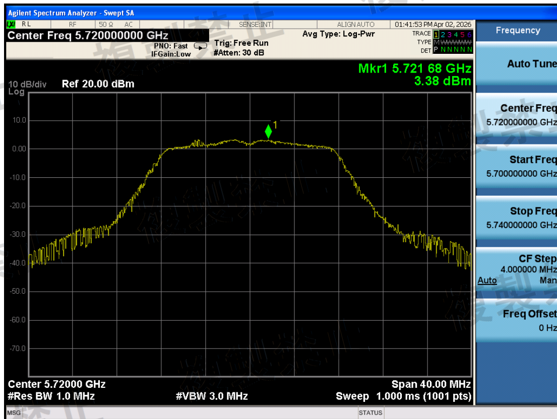
W56\Antenna Power Error\802.11a\1-5720-TX0-N
