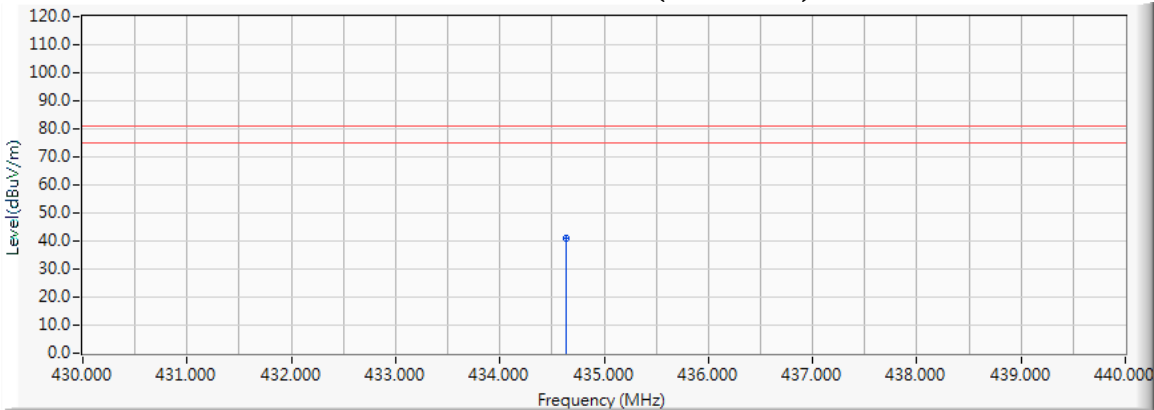
HORIZONTAL_Y- Axis (AVERAGE)
