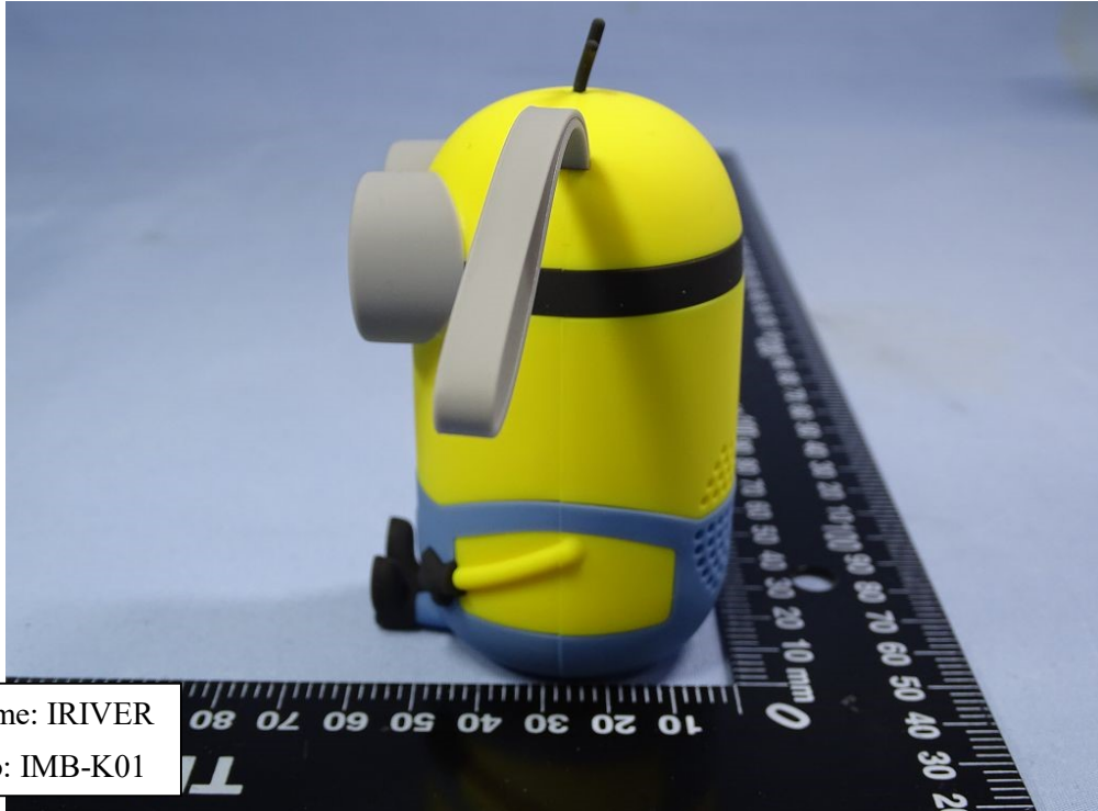
(12) EUT Photo
