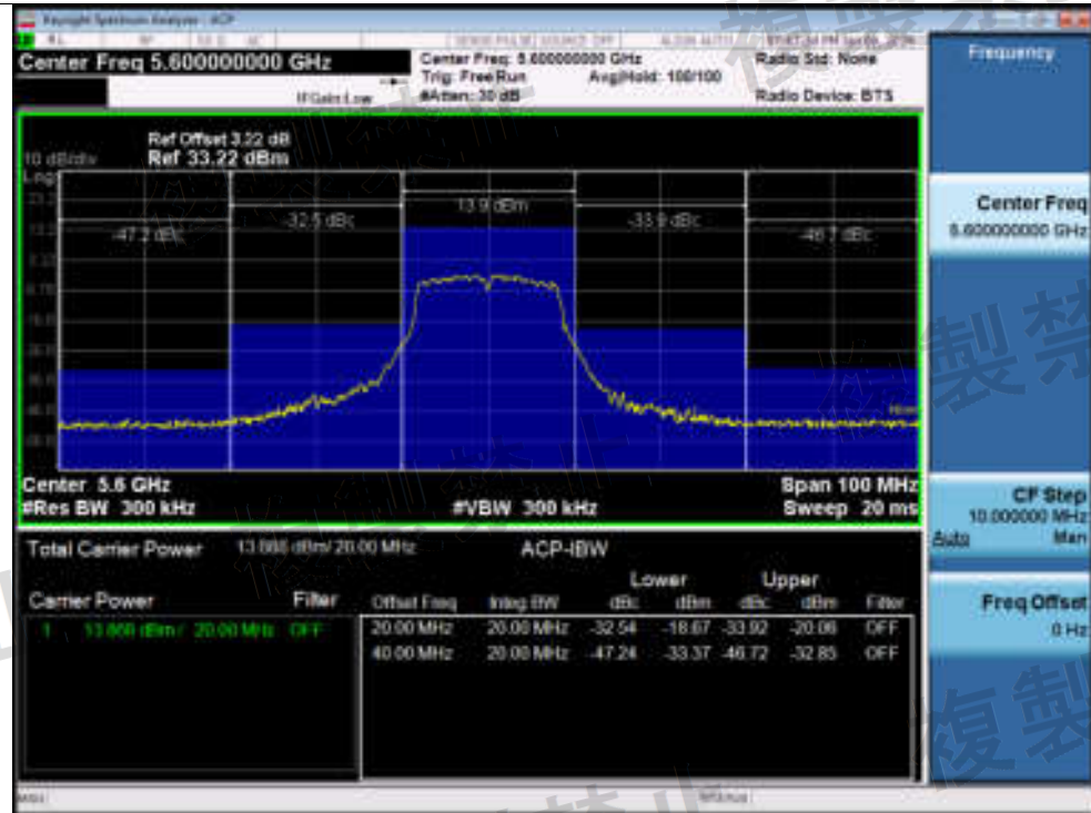
ACEP NVNT a 5600MHz
