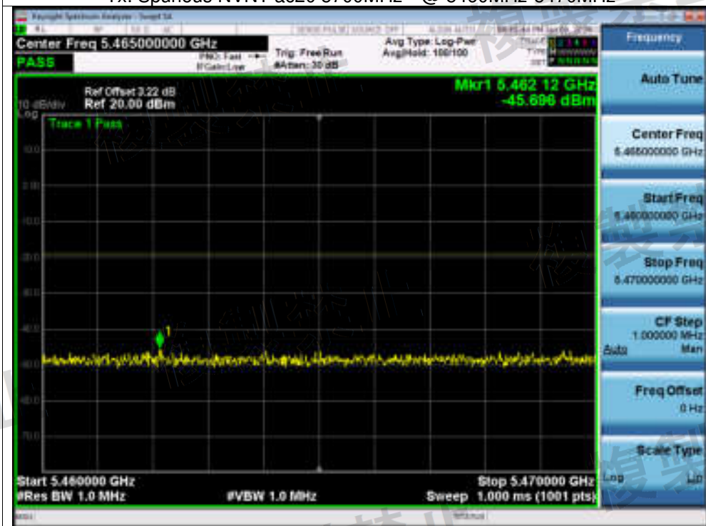
Tx. Spurious NVNT ac20 5700MHz @ 5460MHz-5470MHz
