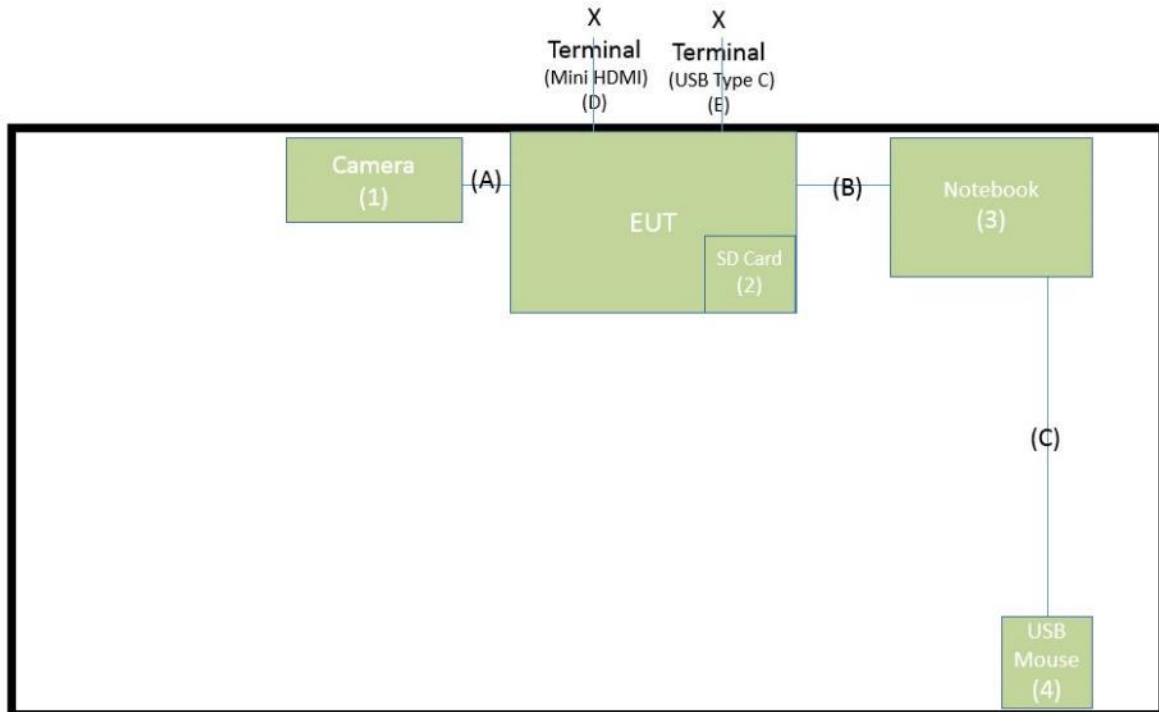
待測物測試配置圖 (Mode1~4)
