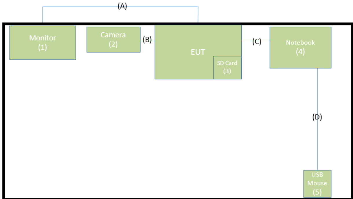
待測物測試配置圖 (Mode5)
