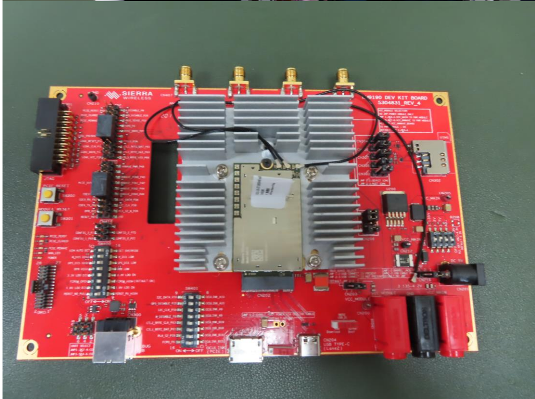
EUT 近照
