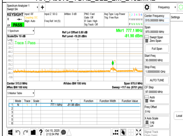
RX Below 1GHz BLE 125k 2402MHz
