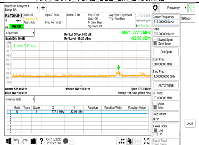
RX Below 1GHz BLE 125k 2480MHz
