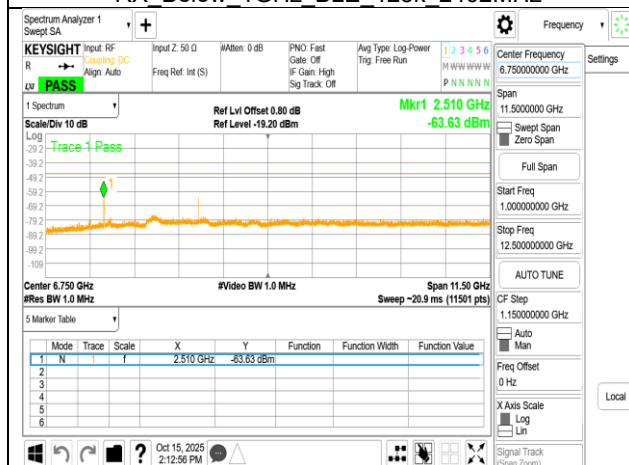
RX Above 1GHz BLE 125k 2402MHz
