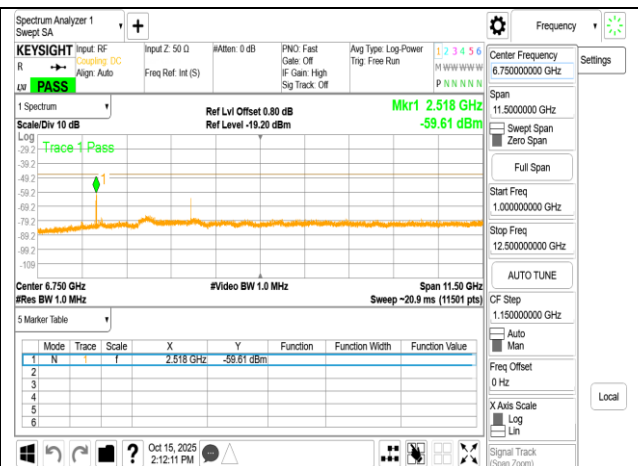
RX Above 1GHz BLE 2M 2480MHz
