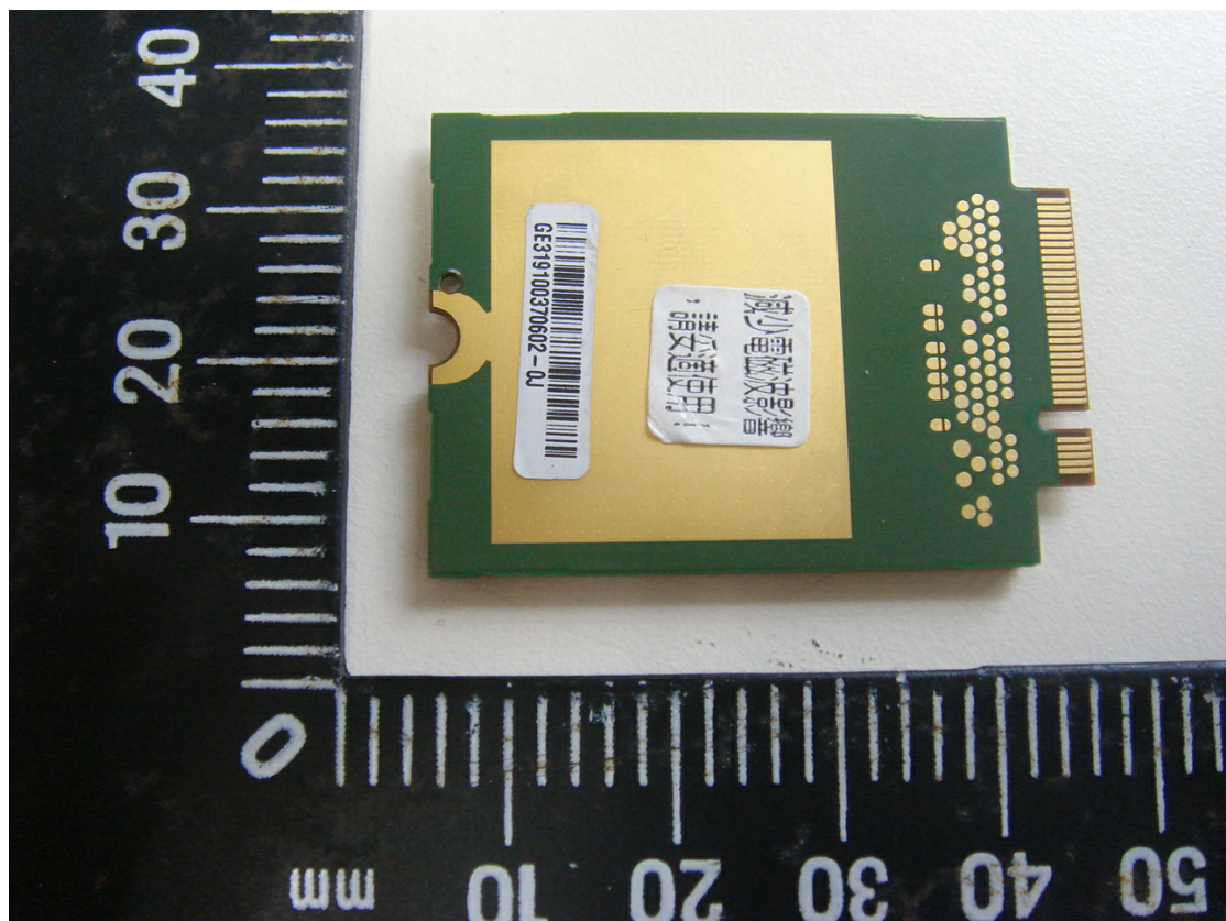
AirPrime MC7330 背面照
